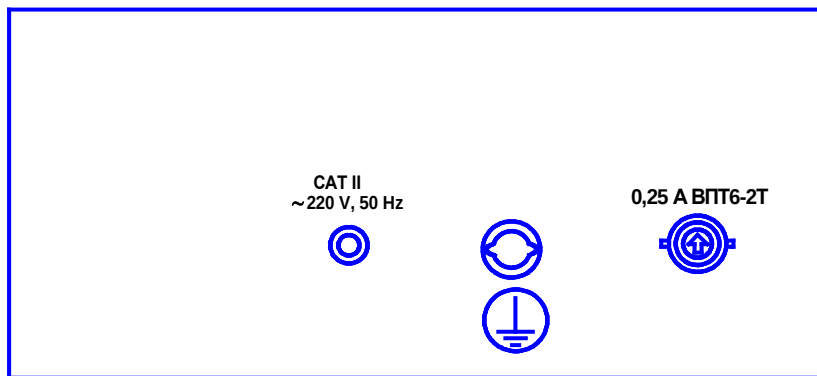
Рисунок 3.2 Измеритель ЦР0200 (задняя панель)
