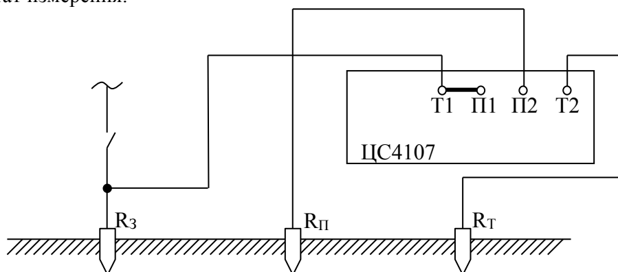
Рисунок 2.4 – Трехпроводная схема подключения измерителя
