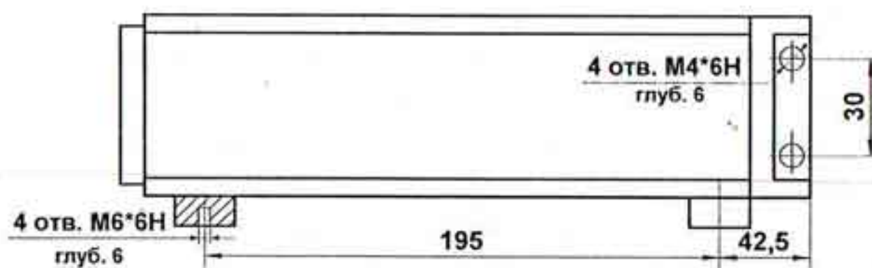
Вид А
