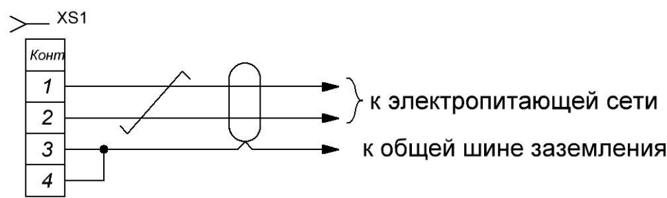
XS1 - соединитель ОНЦ-РГ-09-4/14-Р12 (2РМ14КПН4Г1В1)
