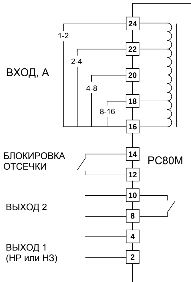
А) PC80M-1...5
