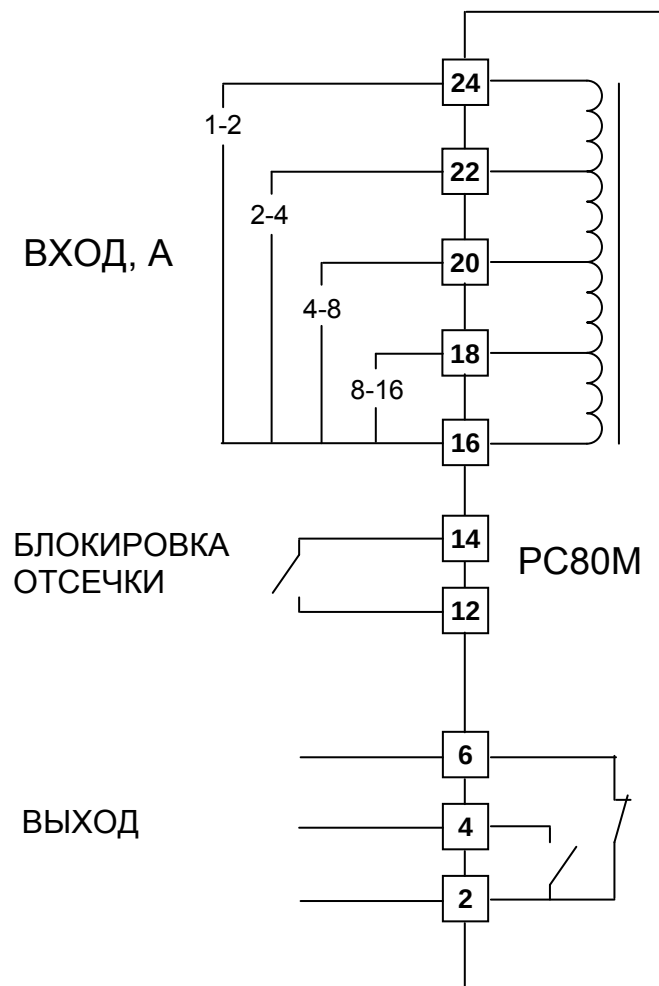
Б) PC80M-6
