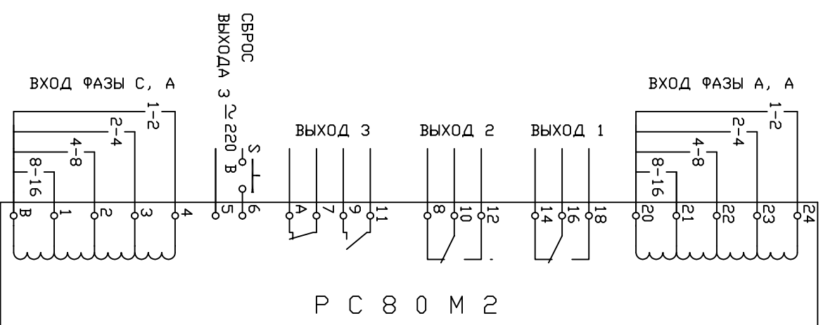
СХЕМА ПОДКЛЮЧЕНИЯ РС80М2-17
