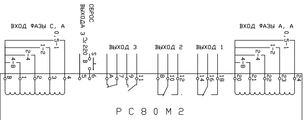
СХЕМА ПОДКЛЮЧЕНИЯ РС80М2-16
