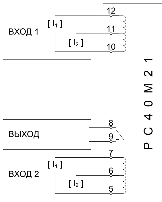
Схема подключения РС40М21(i)
