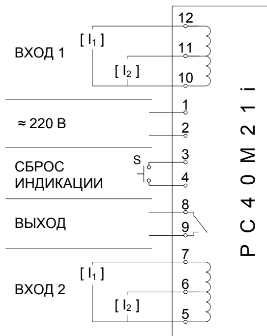
Схема подключения РС40М21(i)
