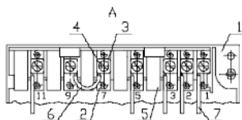
Рис.2 Вариант внутреннего подключения
