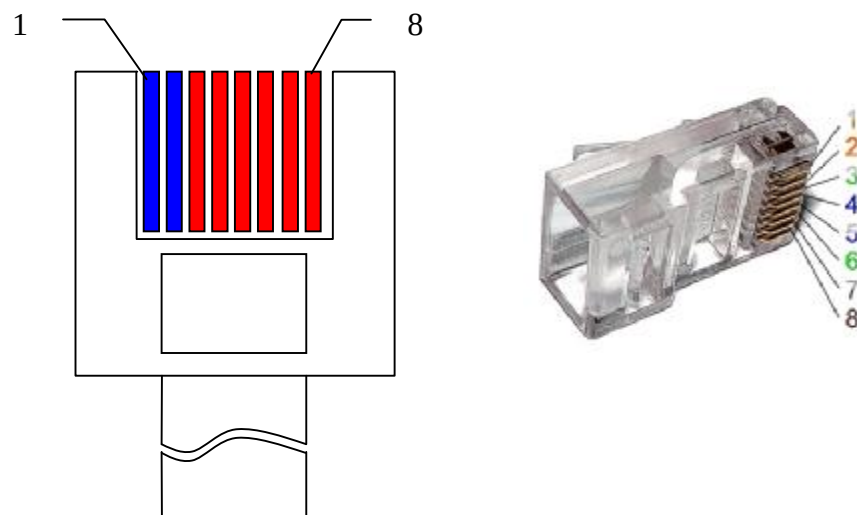
Рисунок 1.4 – Цоколевка разъема RJ-45 (вид со стороны контактов)
