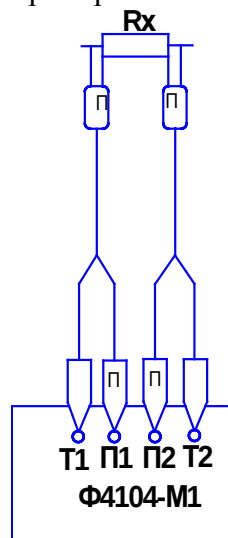
Рисунок 6.1 - Схема измерения сопротивления с исключением влияния соединительных проводов
