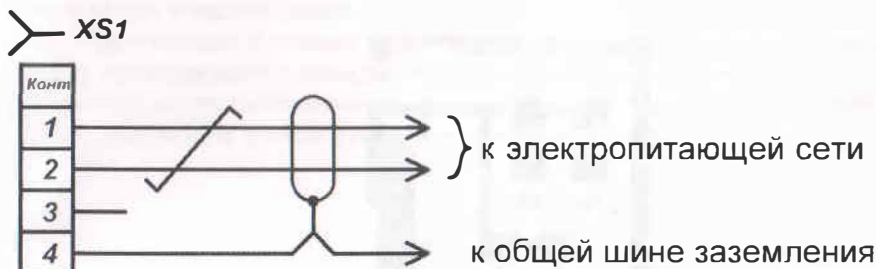
Схема сетевого кабеля
