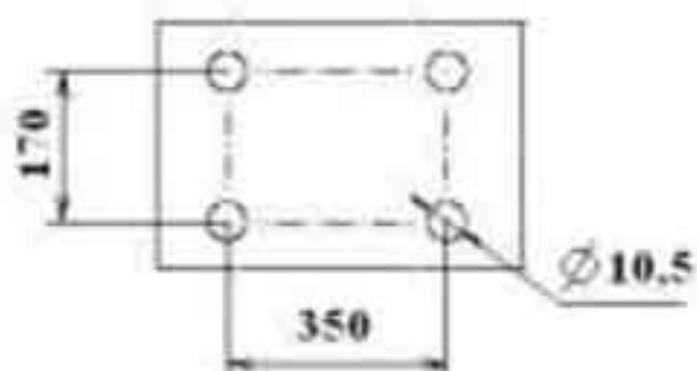
Вид А
