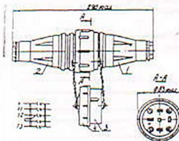
Рис. 1 Соединитель штепсельный СП 063 Габаритные и установочные размеры, основные электрические соединения
