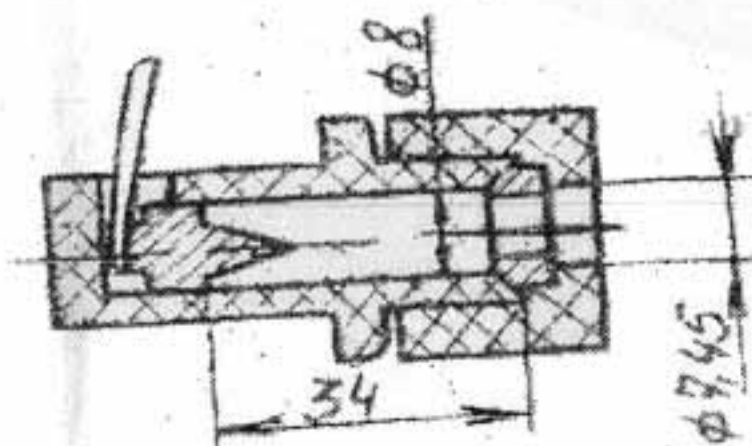
Присоединение нагрузки
