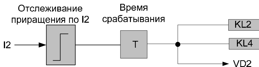
Рис.2. – алгоритм работы по каналу I2
