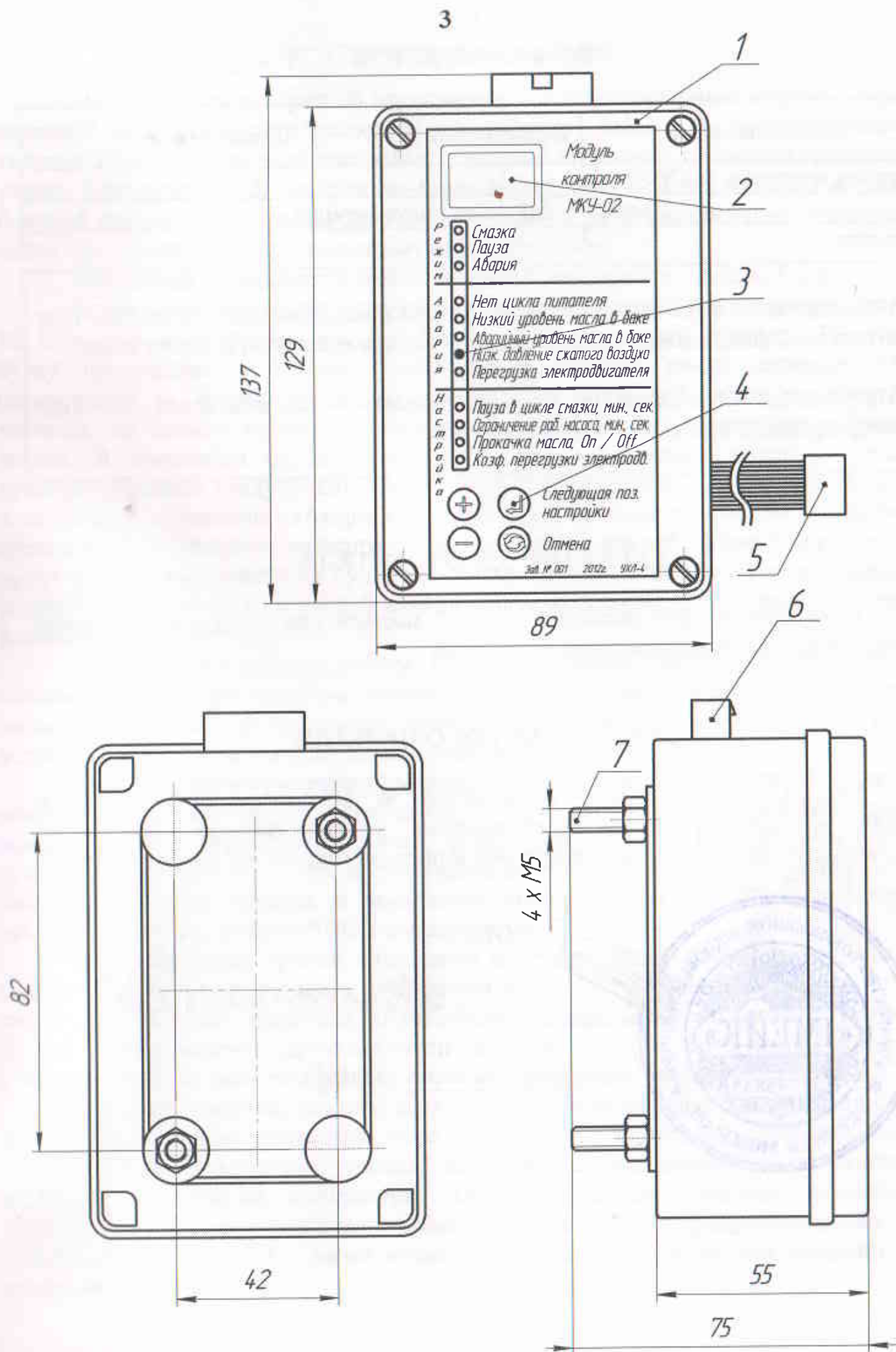
Рисунок 1 - Модуль контроля MKU-02
