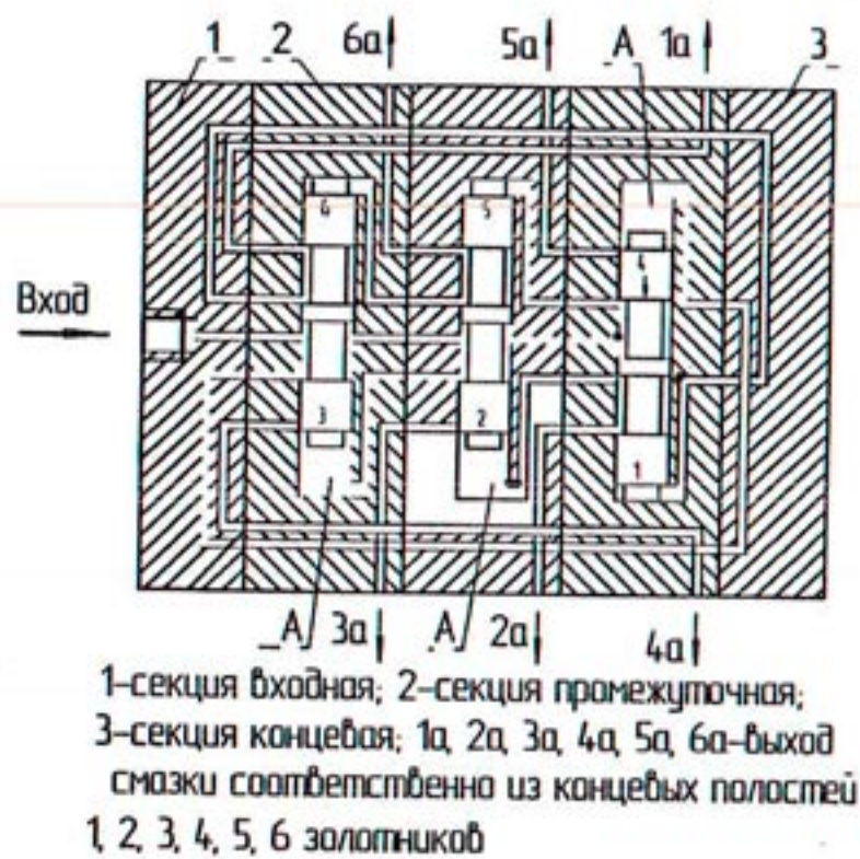
Рисунок 5-Схема работы питателя
