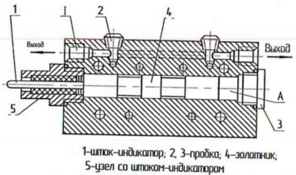
Рисунок 6-Секция промежуточная со штоком-индикатором
