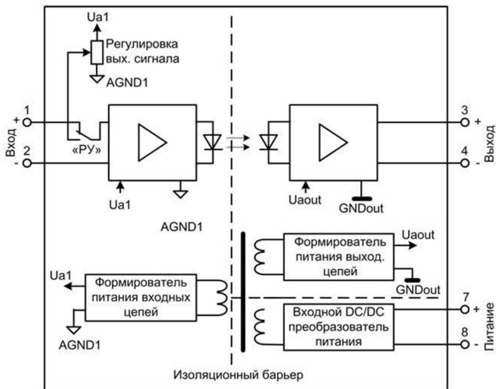
Рис. 4.1 Функциональная схема преобразователя
