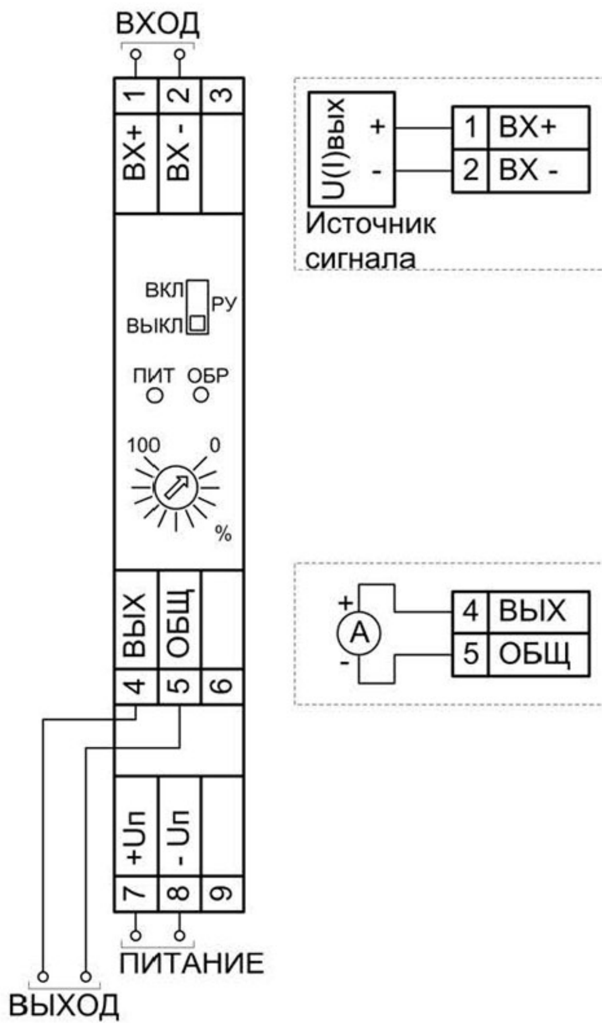
Рис. 4.2 Схема подключения преобразователя
