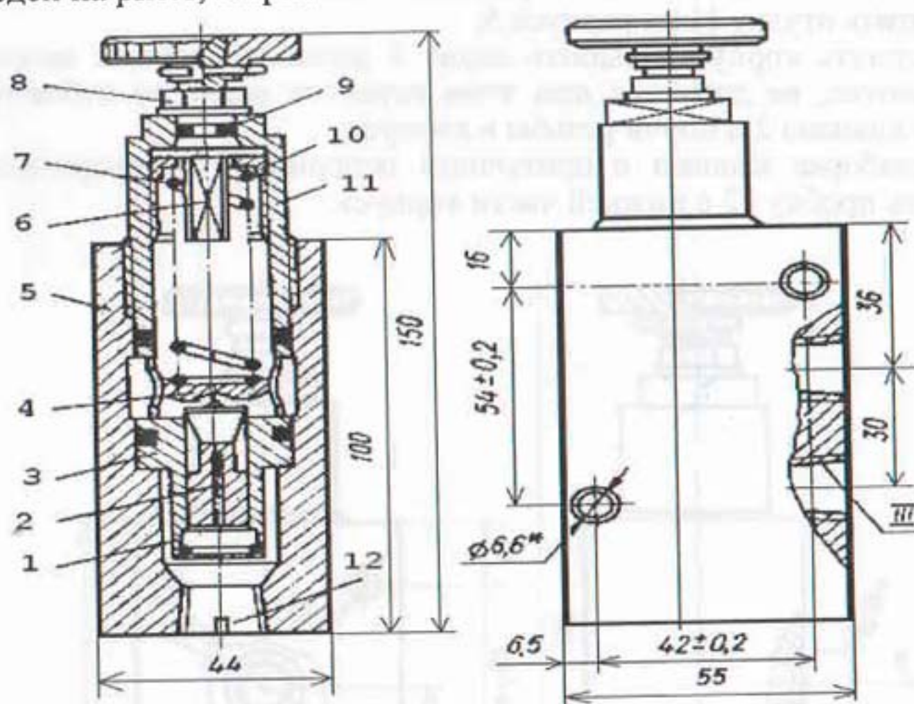
Рис.1. Клапан предохранительный СКП-12/:
