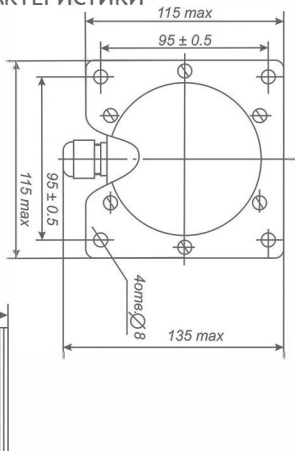
Габаритные и установочные размеры
