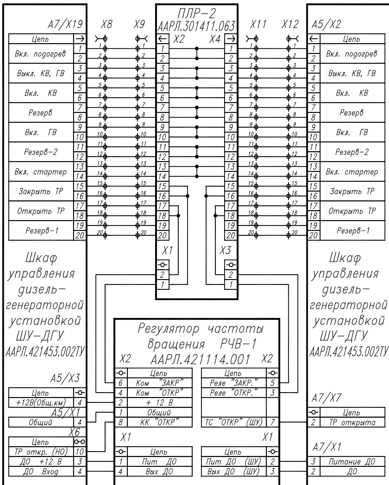
Рисунок 4 - Схеме стыковки РЧВ с ШУ-ДГУ.
