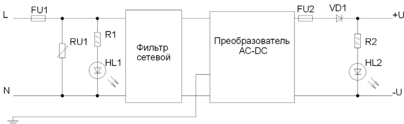
Рисунок 1.2 – Схема структурная электрическая блока БП-30-2к
