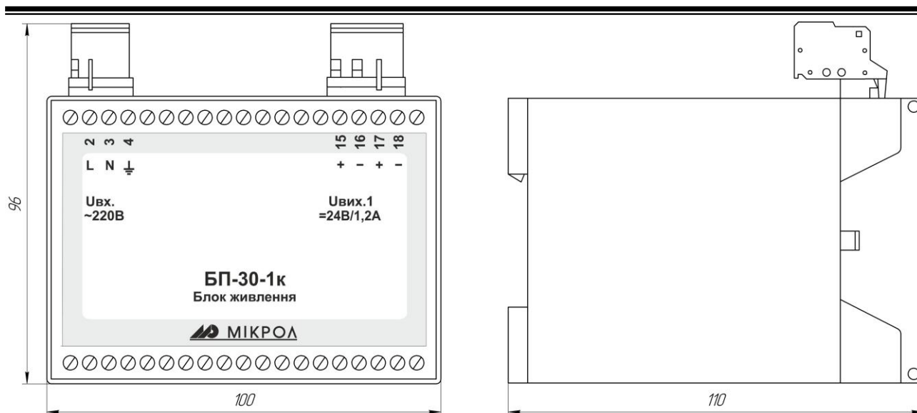
Рисунок 1.1 – Внешний вид и габаритные размеры БП-30-1к
