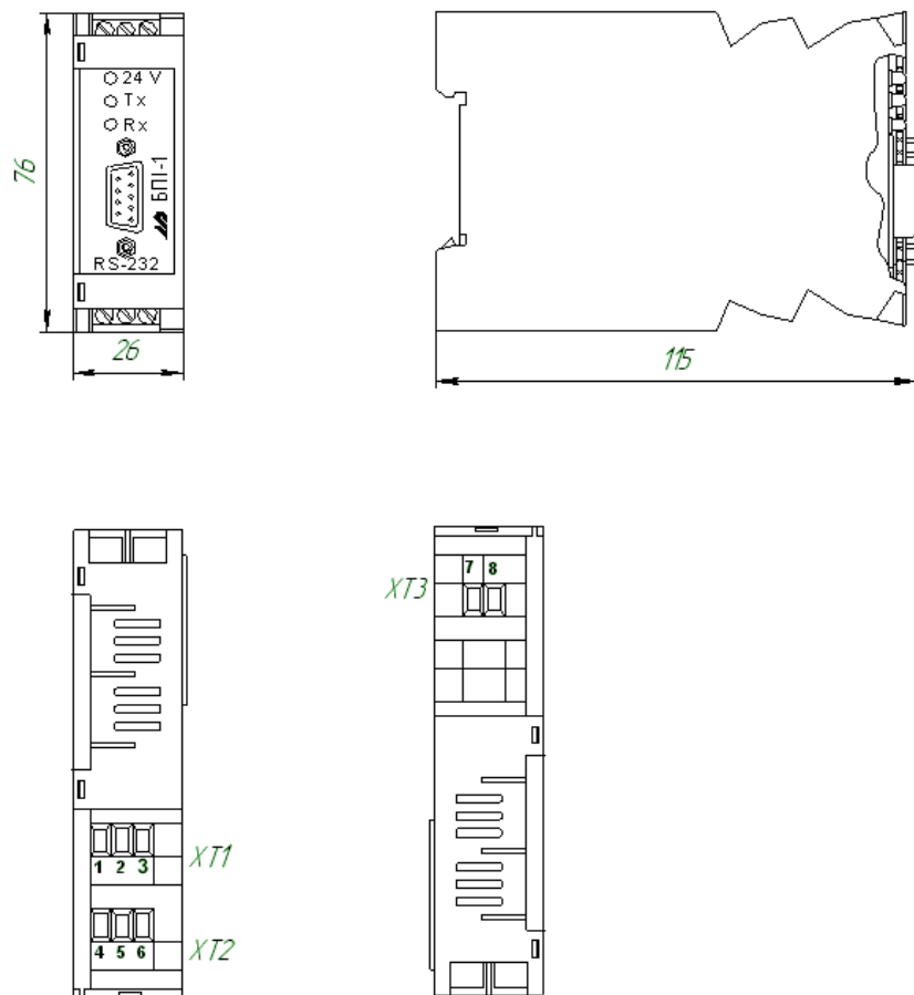
Рисунок Б.1 Габаритные соединительные размеры блока БПИ-1
