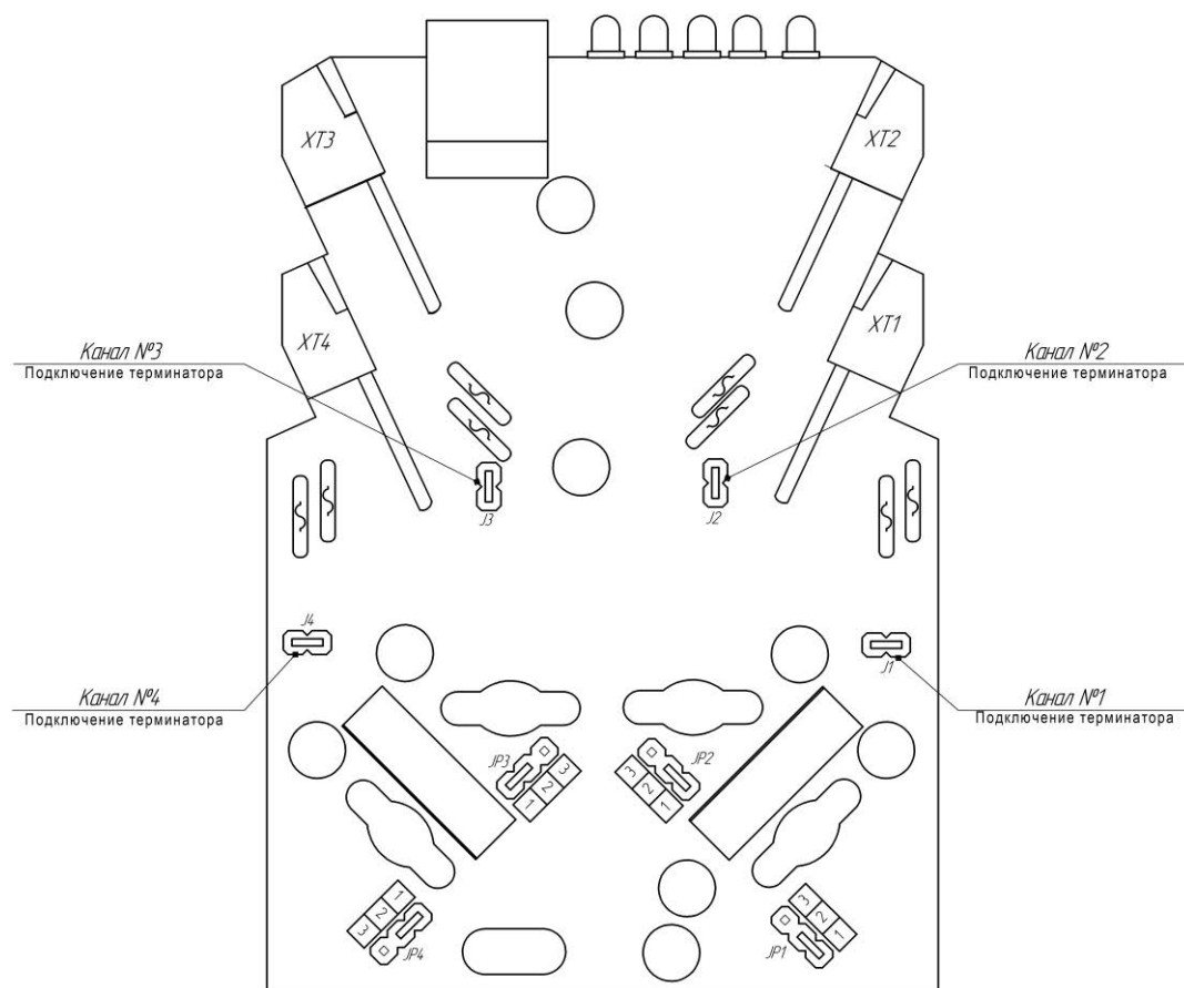
А.2 Расположение перемычек блока БПИ-452.
