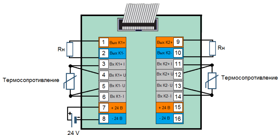
Рисунок 4.3 Схема электрических подключений к КБЗ-16-11
