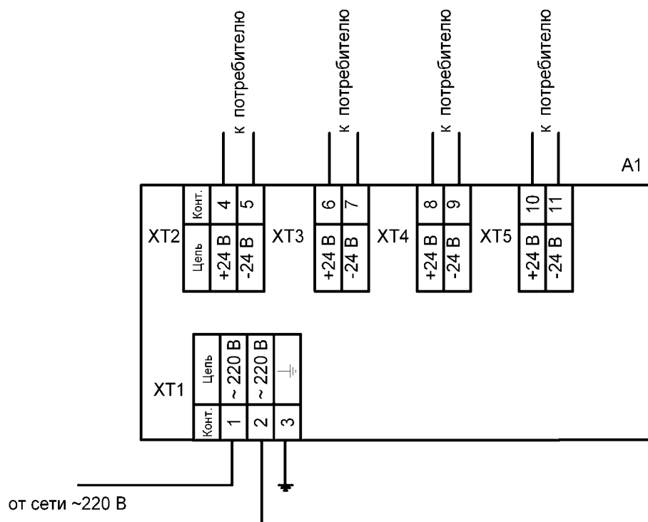
А1 - блок питания БПС24-4к
