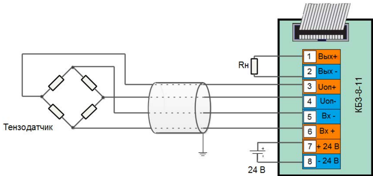
Рисунок В.1 - Схема внешних соединений одного тензодатчика БПТ-2 с использованием KB3-8-11
