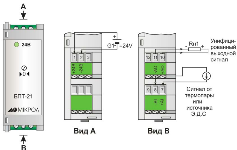
Рисунок 4.2.3 - Схема электрических подключений блока БПТ-21
