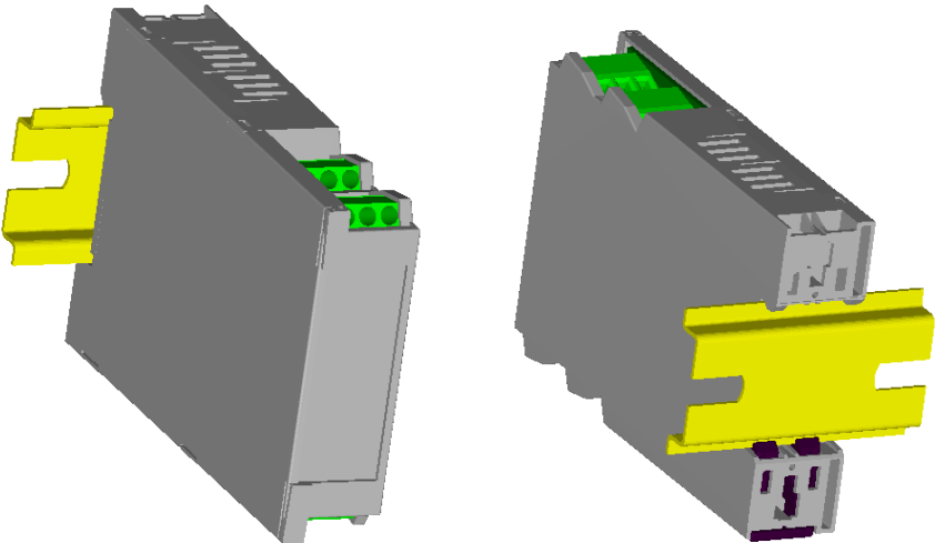
Рисунок 4.2.1 - Схема крепления блока БПТ-22 на DIN-рельсе
