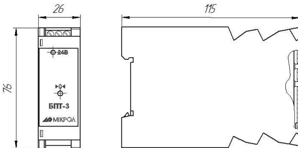
Рисунок 1.4 - Внешний вид и габаритные размеры БПТ-3
