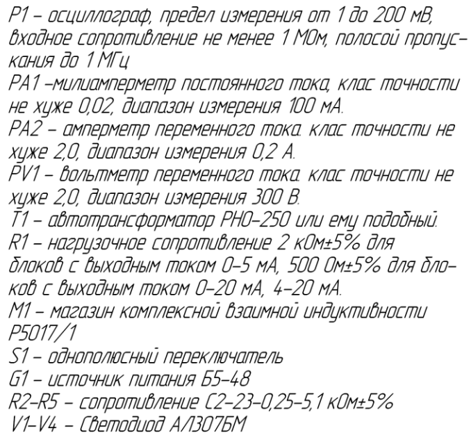
Рисунок Б.4 – Схема подключения прибора для проведения наладки
