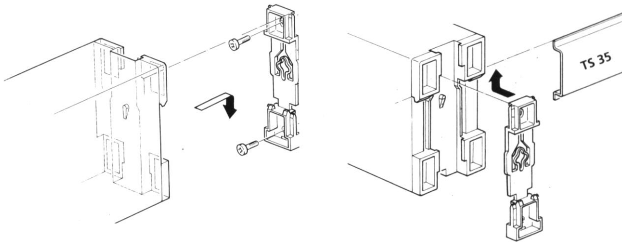
Вариант крепления на плоскость
