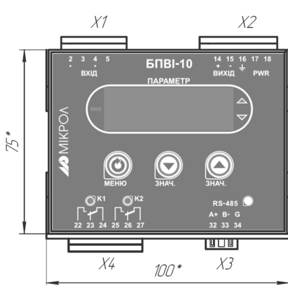
Рисунок А.1 – Внешний вид передней панели преобразователя БПВІ-10
