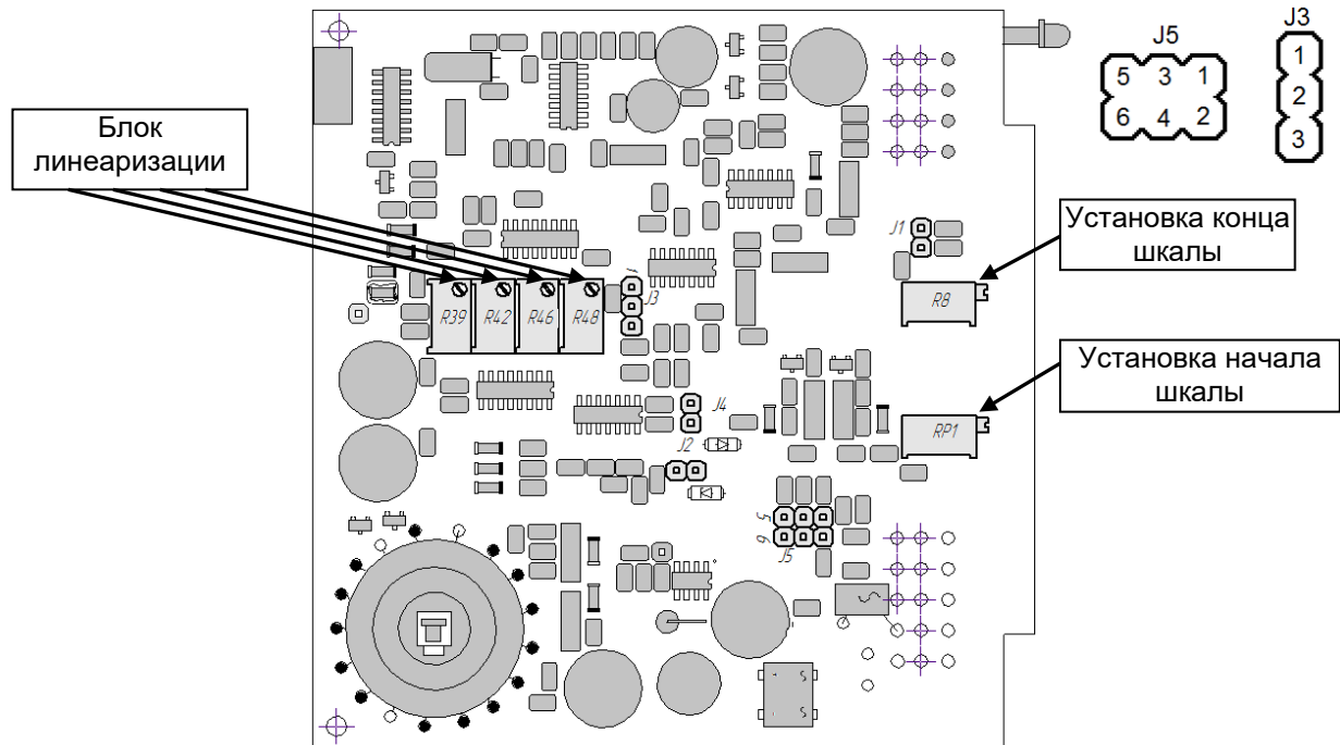
Рисунок 5.1.1 - Схема расположения органов регулирования и элементов настройки БПВ1-10
