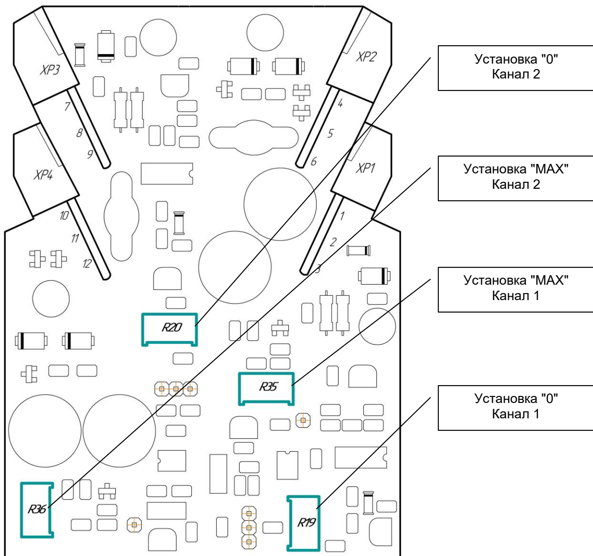
Рисунок 4.1 – Схема расположения элементов настройки БРГ-412
