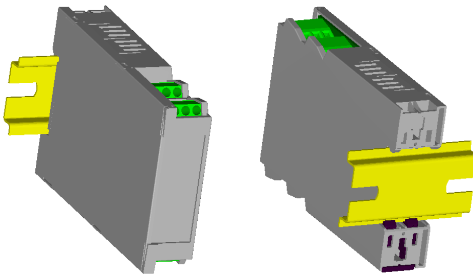
Рисунок 3.1 – Схема крепления блока БРГ-412 на щит
