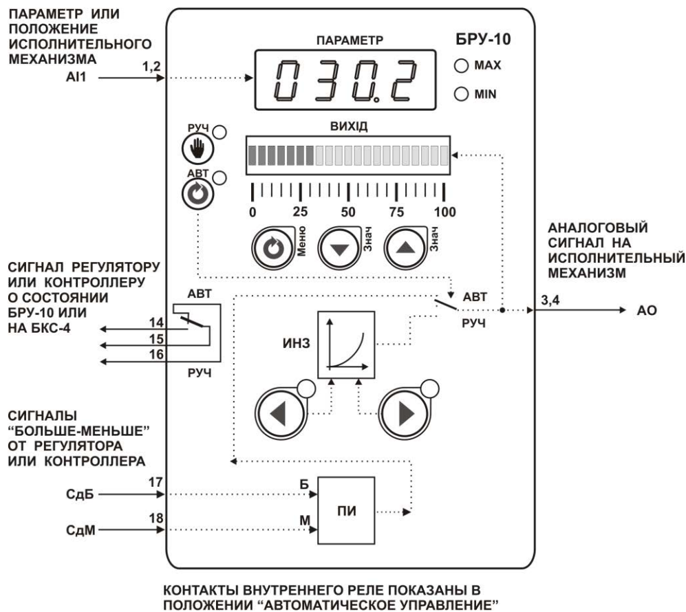
Рисунок 7.10.1 - Блок-схема режима 9
