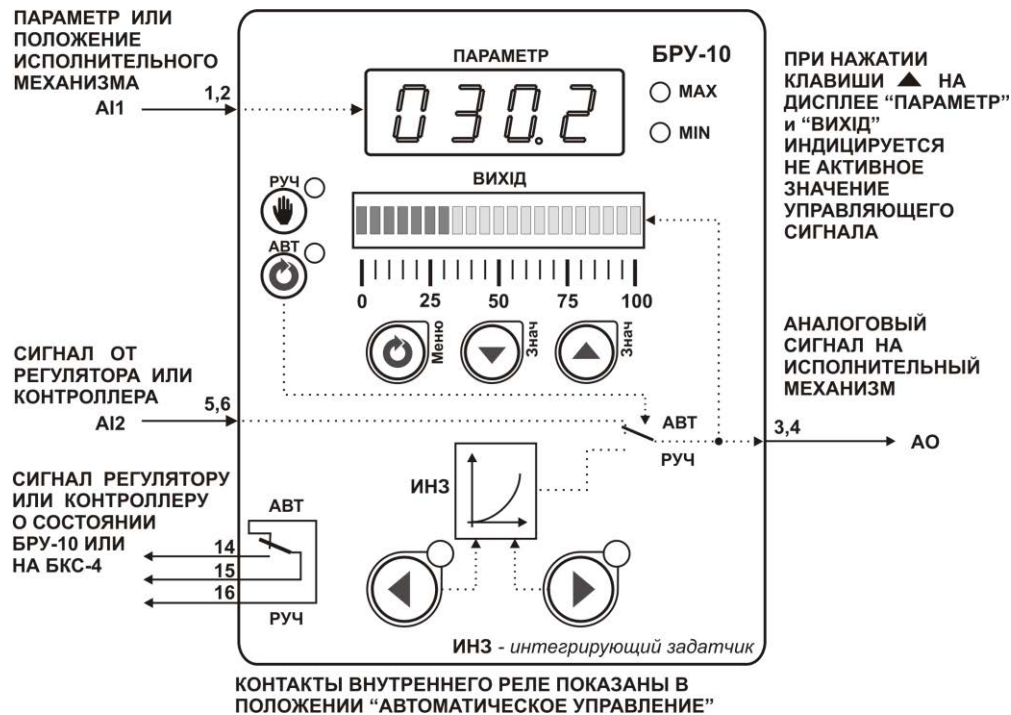
Рисунок 7.12.1 - Блок-схема режима 11
