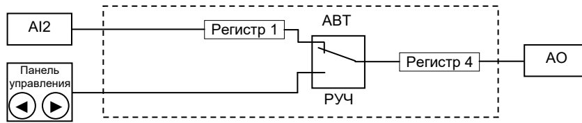
Рисунок 7.2.2 - Функциональная схема балансировок режима 1
