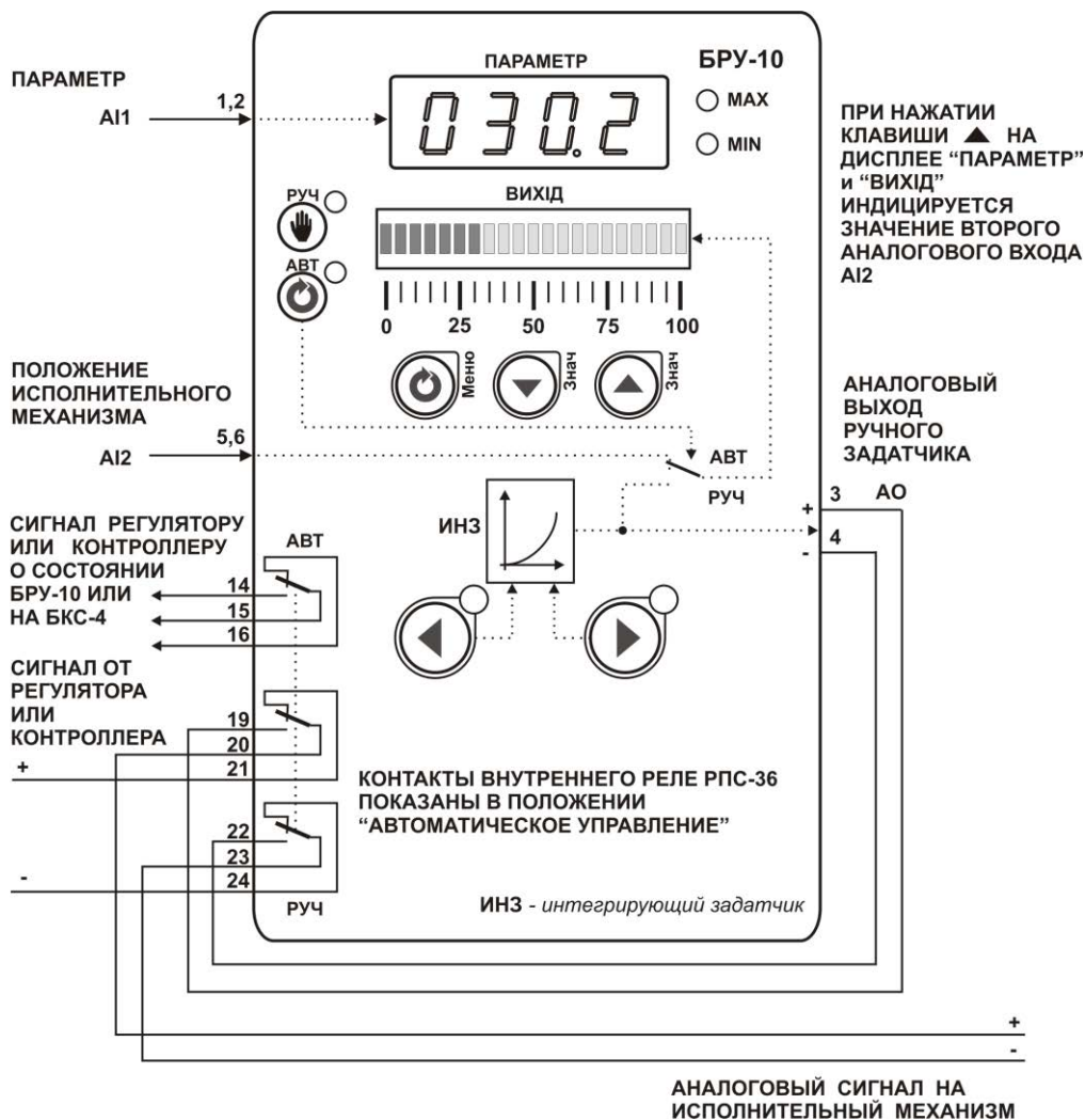
Рисунок 7.2.1 - Блок-схема режима 1
