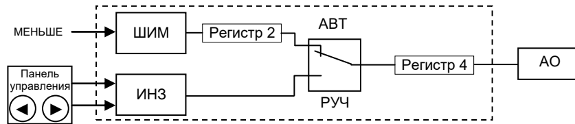
Рисунок 7.6.2 - Функциональная схема балансировок режима 5
