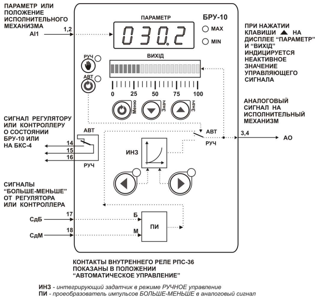
Рисунок 7.5.1 - Блок-схема режима 4
