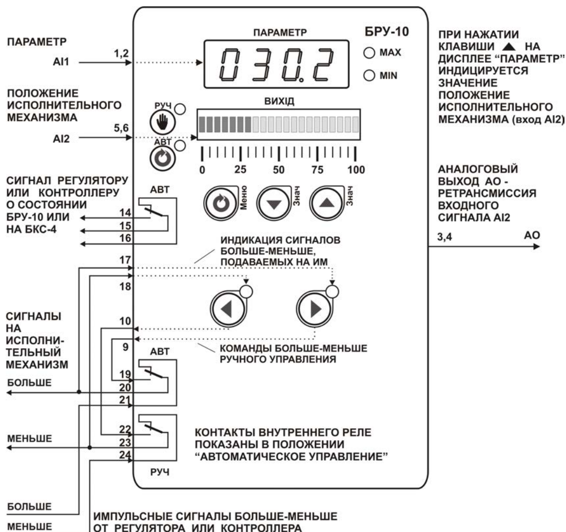
Рисунок 7.4.1 - Блок-схема режима 3
