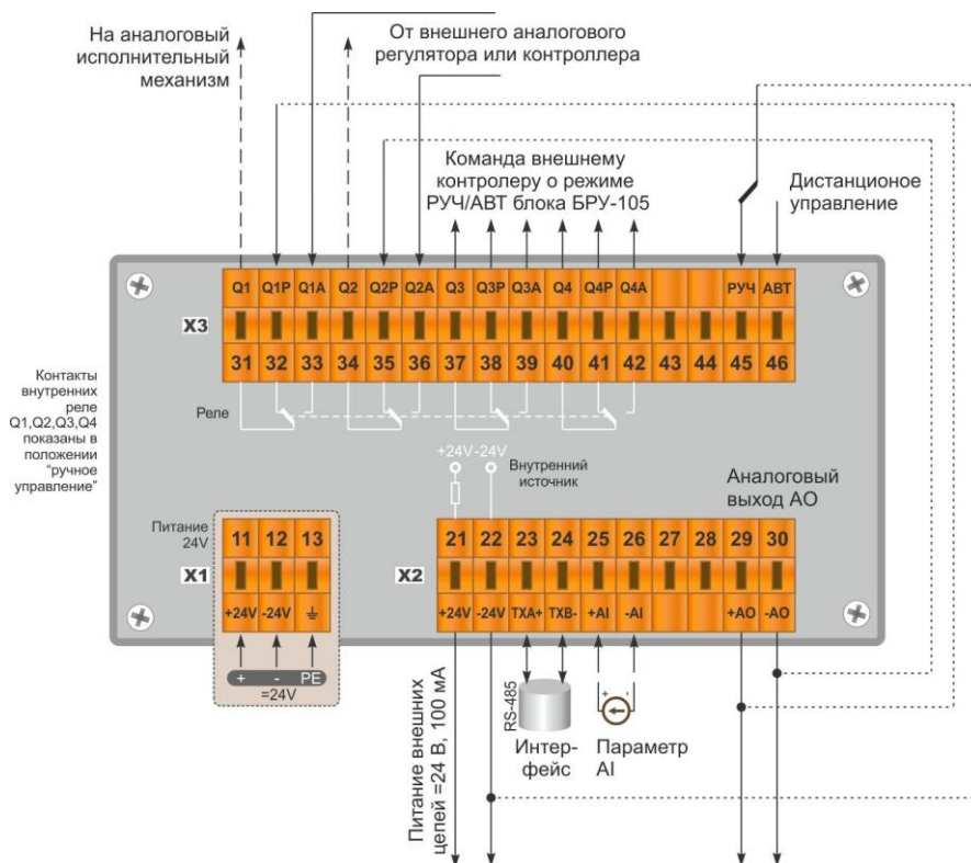
Рисунок Б.2 – Схема внешних соединений блока ручного управления БРУ-17
