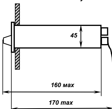
Вид сбоку
