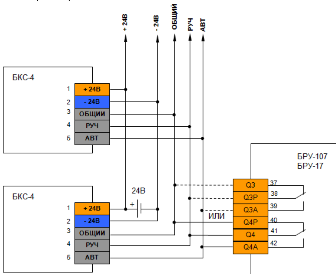
Рисунок Б.3 - Схема подключения блока коммутации сигналов БКС-4 к БРУ-107 (БРУ-17)
