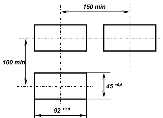
Разметка отверстий на щите
