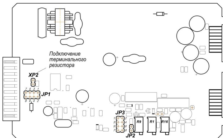
Рисунок 4.2 – Положение переключателей на плате входов БРУ-107
