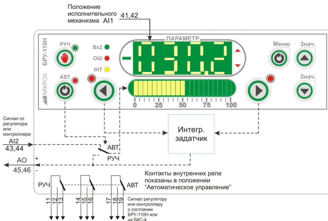
Рисунок 4.23 - Блок-схема режима 11
