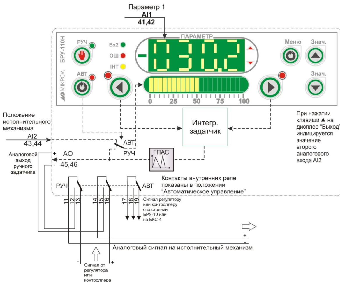
Рисунок 4.22 - Блок-схема режима 10
