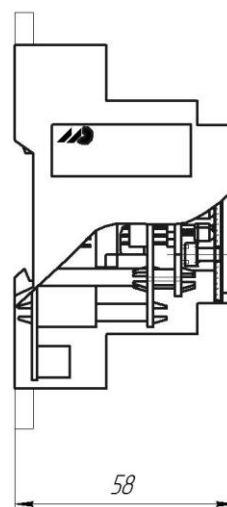
Вид сбоку
