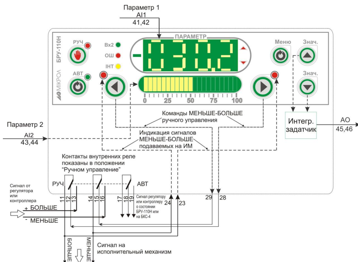
Рисунок 4.17 - Блок-схема режима 7
