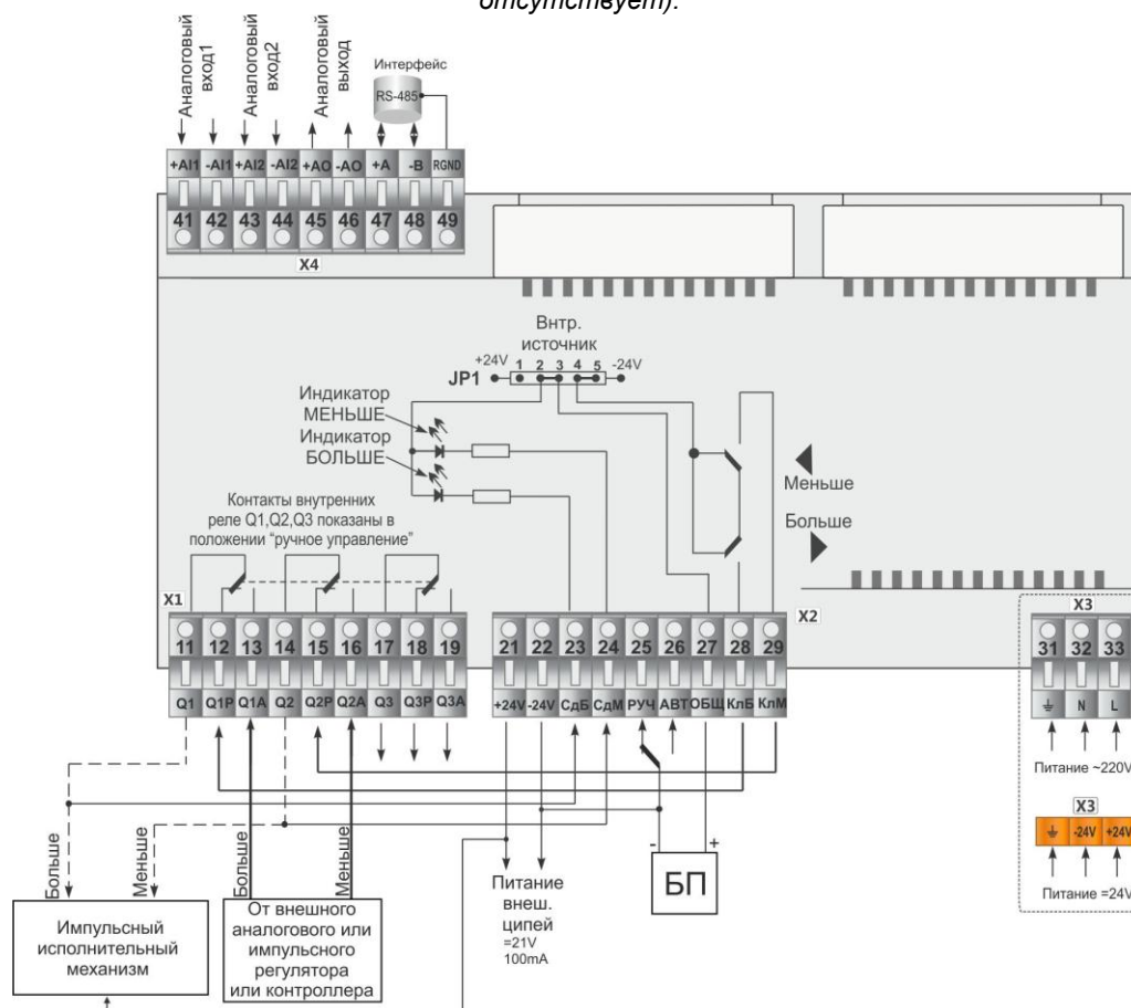
Рисунок. Б.5 – Подключение индикаторов БОЛЬШЕ-МЕНЬШЕ блока БРУ-110Н через внешний источник питания
