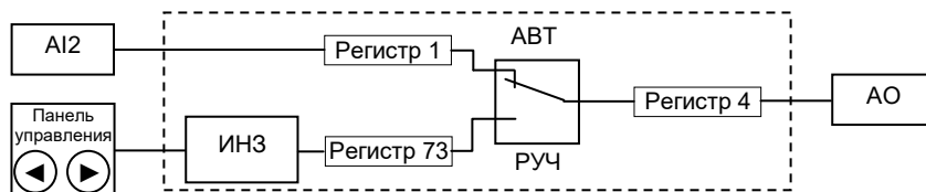
Рисунок 4.24 - Функциональная схема балансировки режима 11
