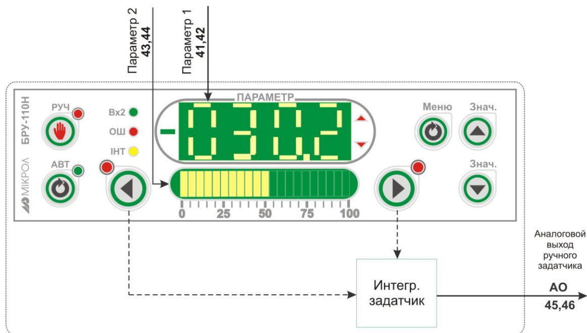
Рисунок 4.7 - Блок-схема режима 0
