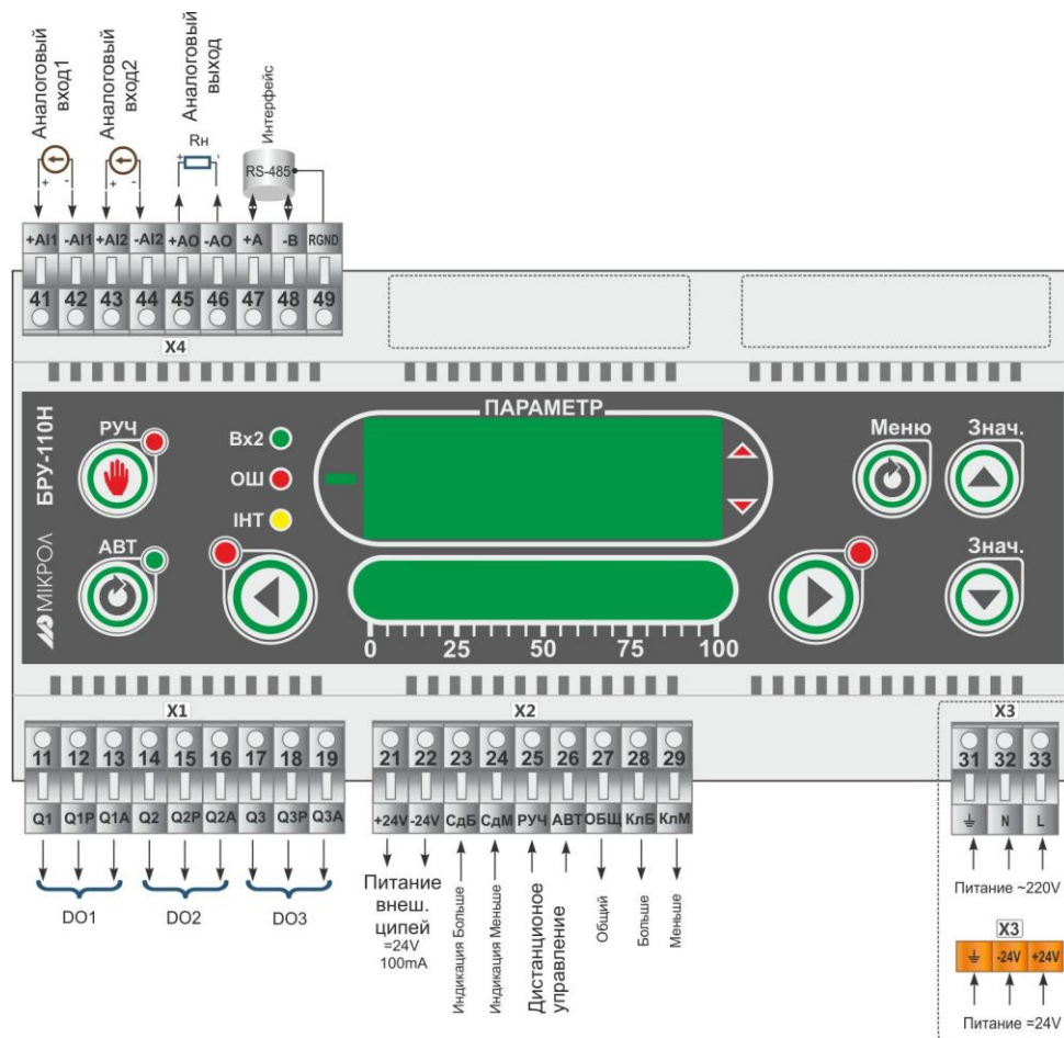
Рисунок Б.1 - Подключение к блоку ручного управления БРУ-110Н
