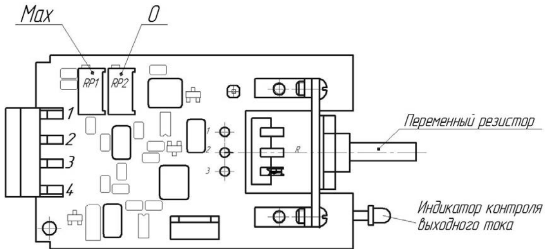
Рисунок 2- Расположение органов регулировки выходного сигнала блока ручного управления БРУ-420
