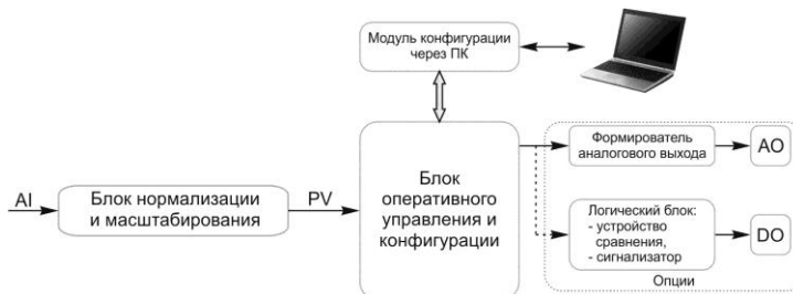
Рисунок 3.3 - Функциональная схема вольтметра ИПМ-1
