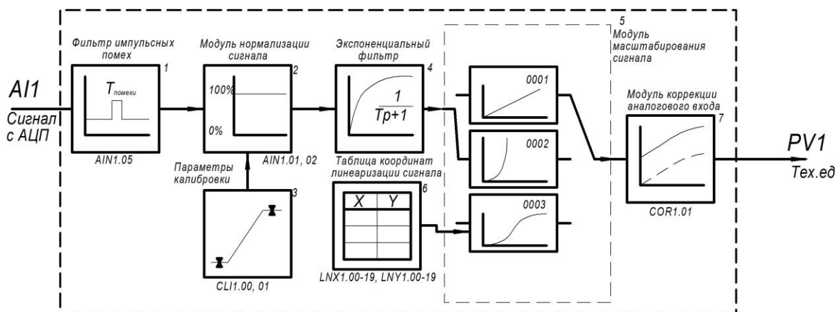
Рисунок 3.4 – Блок-схема обработки аналогового входа
