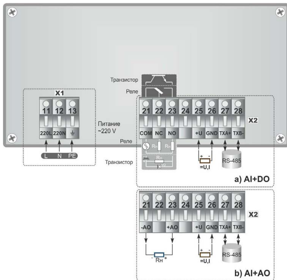
Рисунок Б.1 - Подключение внешних цепей к вольтметру ИПМ-1: а) подключение при условии заказа опции дискретного выхода; б) подключение при условии заказа опции аналогового выхода.
