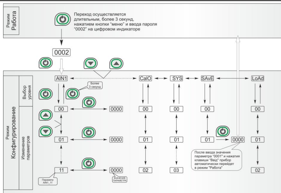
Рисунок 4.1 - Диаграмма уровней конфигурации и настроек
