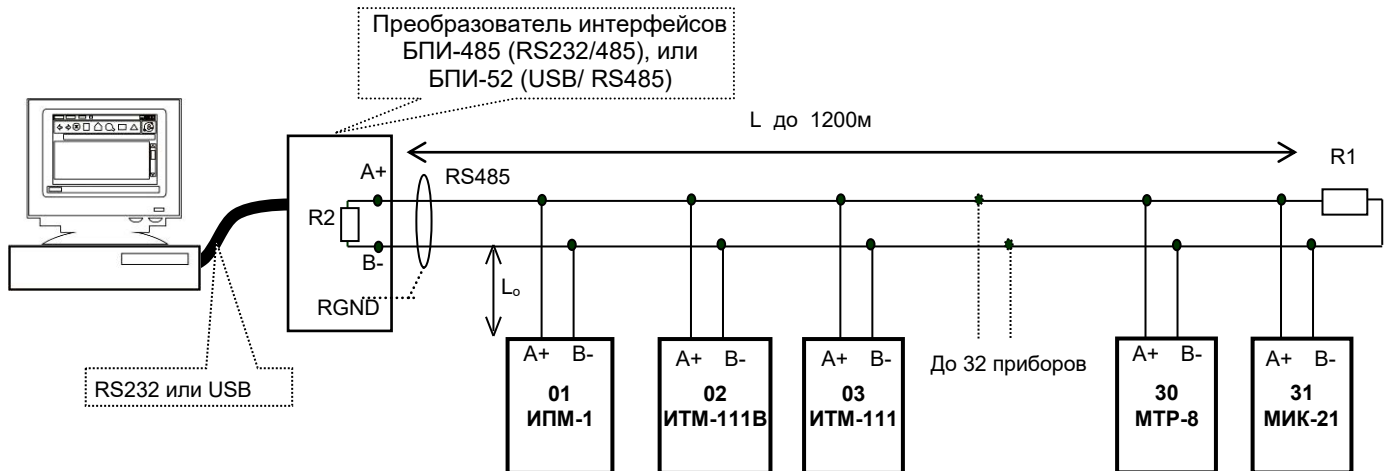
Рисунок Б.3 - Организация интерфейсной связи между компьютером и вольтметрами или контроллерами
