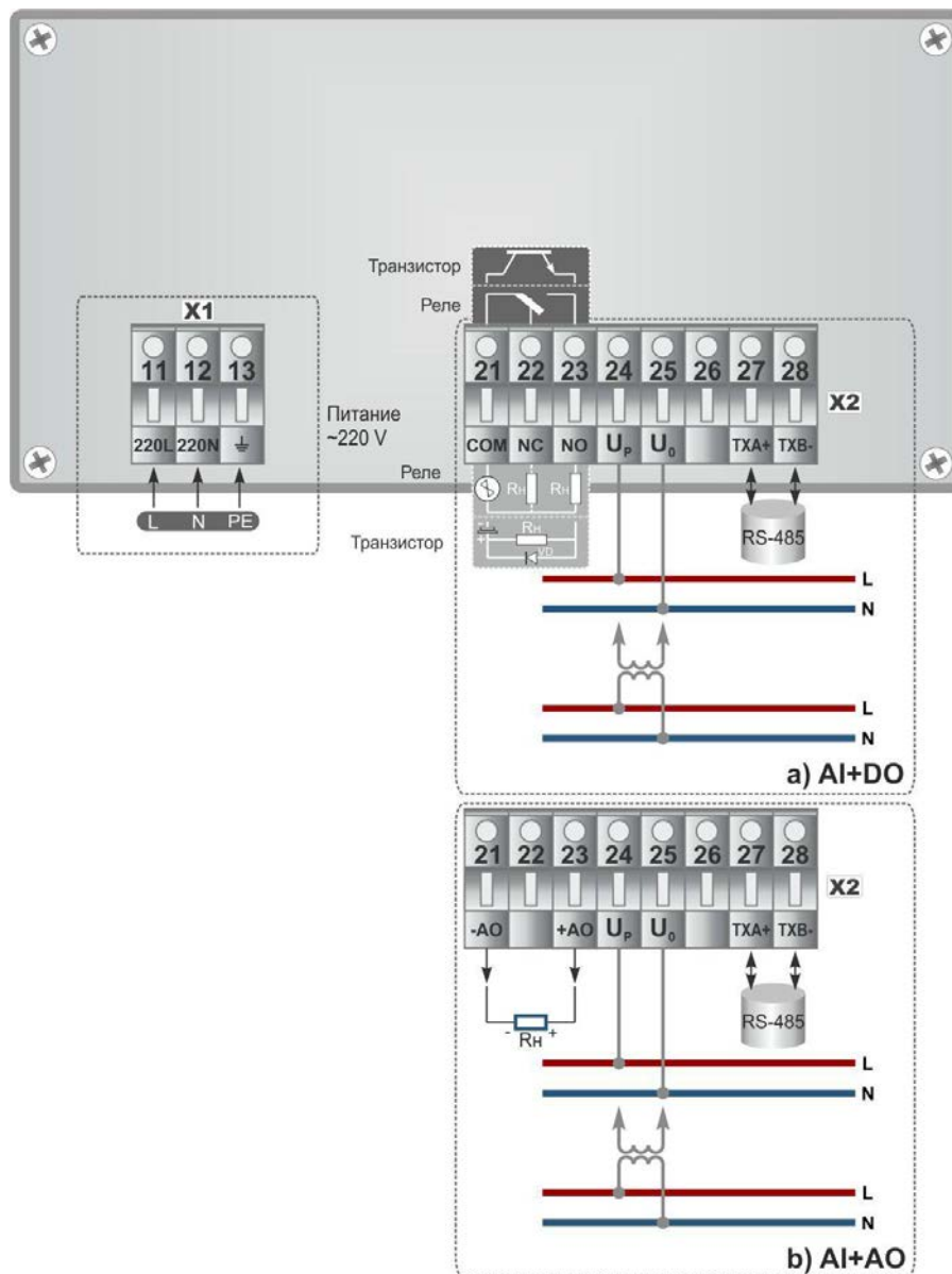
Рисунок Б.1 - Подключение внешних цепей к вольтметру ИПМ-2: а) подключение при условии заказа опции дискретного выхода; б) подключение при условии заказа опции аналогового выхода.
