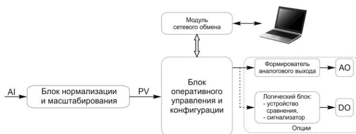
Рисунок 3.3 - Функциональная схема вольтметра ИПМ-2
