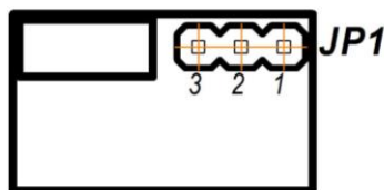
Рисунок 5.1 – Положение перемычек на модуле аналогового выхода
