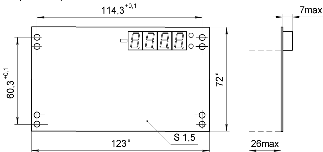
Рисунок А.1.1 – Габаритные размеры ИТМ-1-10
