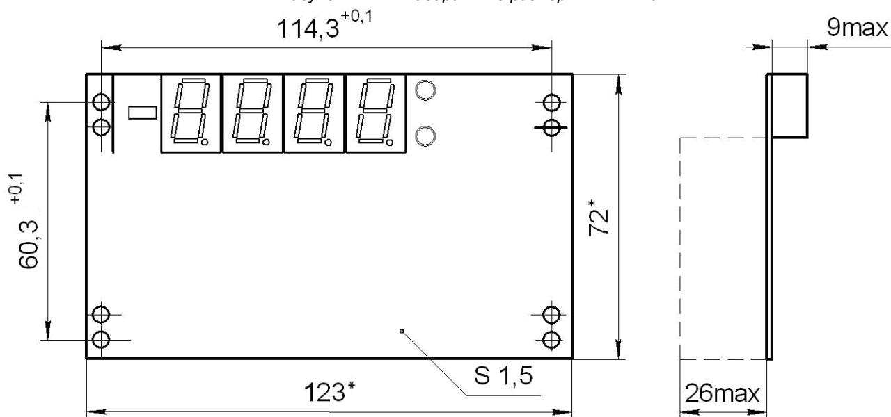
Рисунок А.1.2 – Габаритные размеры ИТМ-1-14
