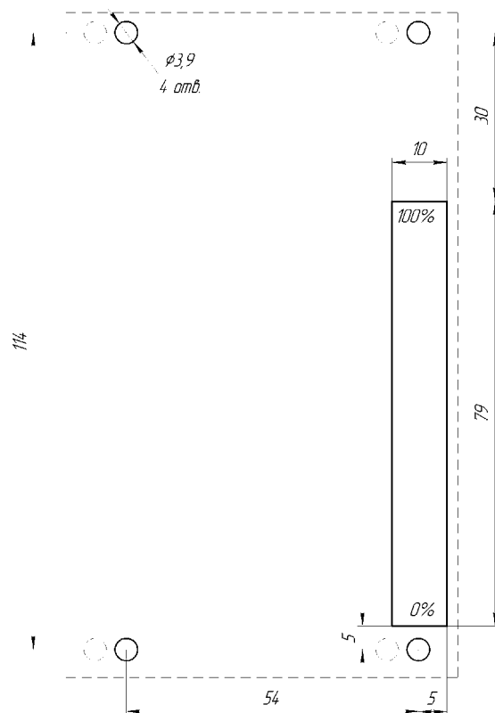
Рисунок А.4 - Рекомендуемый вырез в щите для вертикального положения индикатора ИТМ-1-01-31
