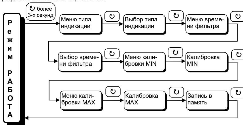
Рисунок 6.3 - Диаграмма уровней конфигурации и настроек.
