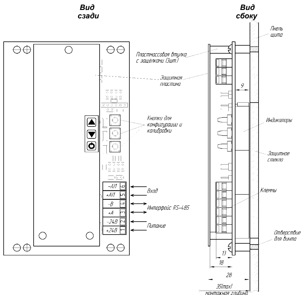
Рисунок А.1 – Габаритные размеры
