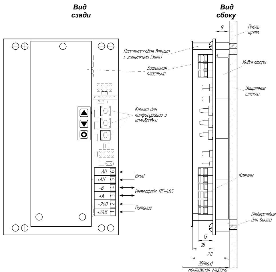
Рисунок А.5 – Габаритные размеры
