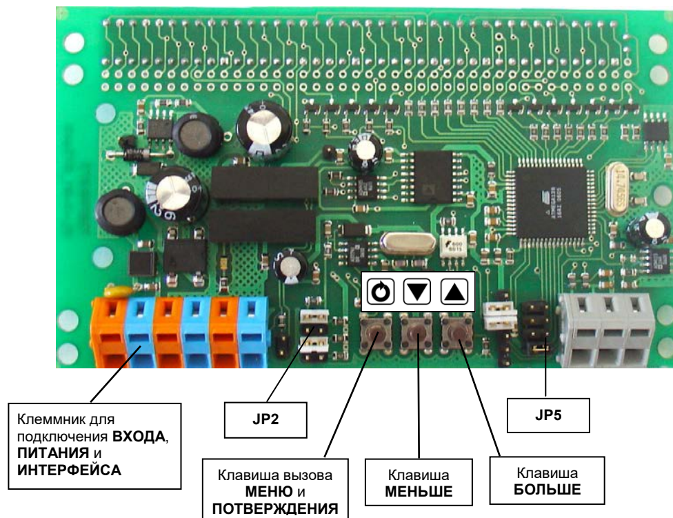
Рисунок 5.2 – Индикатор ИТМ-1-01-41. Вид сзади.
