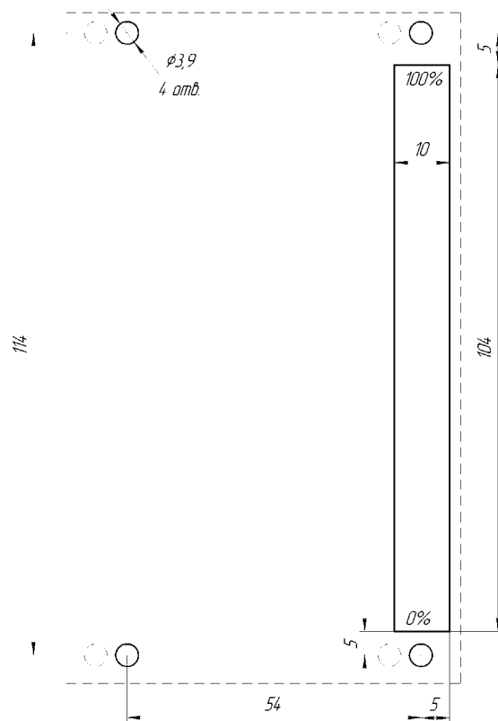
Рисунок А.8 - Рекомендуемый вырез в щите для вертикального положения индикатора ИТМ-1-01-41
