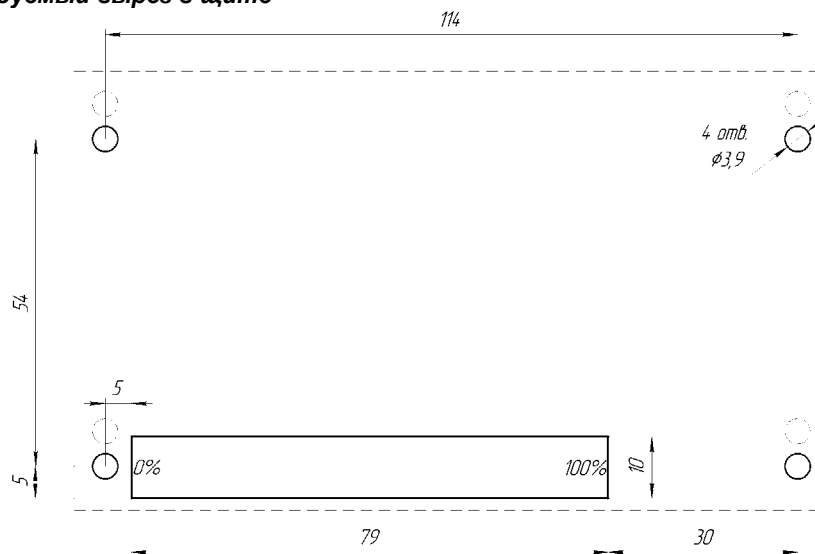
Рисунок А.3 - Рекомендуемый вырез в щите для горизонтального положения индикатора ИТМ-1-01-31
