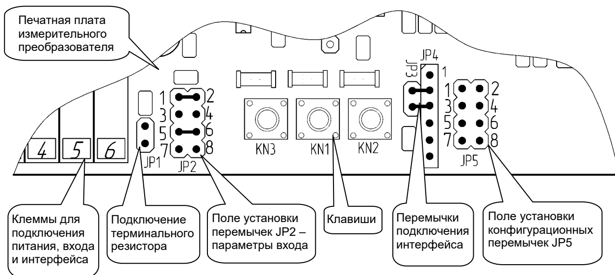
Рисунок 6.2 - Расположение конфигурационных перемычек на плате ИТМ-1-01-31 и ИТМ-1-01-41
