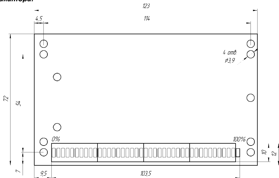
Рисунок А.5 – Габаритные размеры
