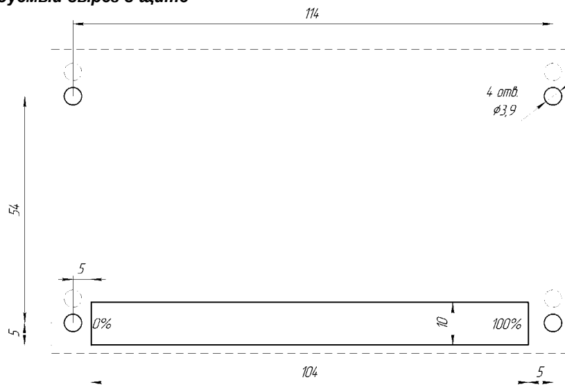
Рисунок А.7 - Рекомендуемый вырез в щите для горизонтального положения индикатора ИТМ-1-01-41
