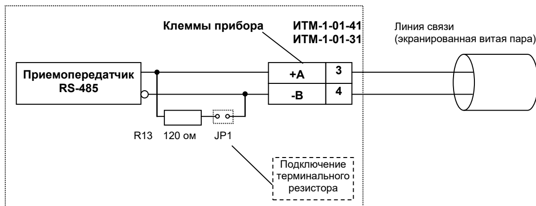
Рисунок Б.2 - Рекомендуемая схема подключения интерфейса RS-485 на индикаторах ИТМ-1-01-31 и ИТМ-1-01-41
