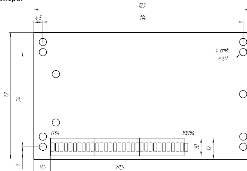
Рисунок А.1 – Габаритные размеры
