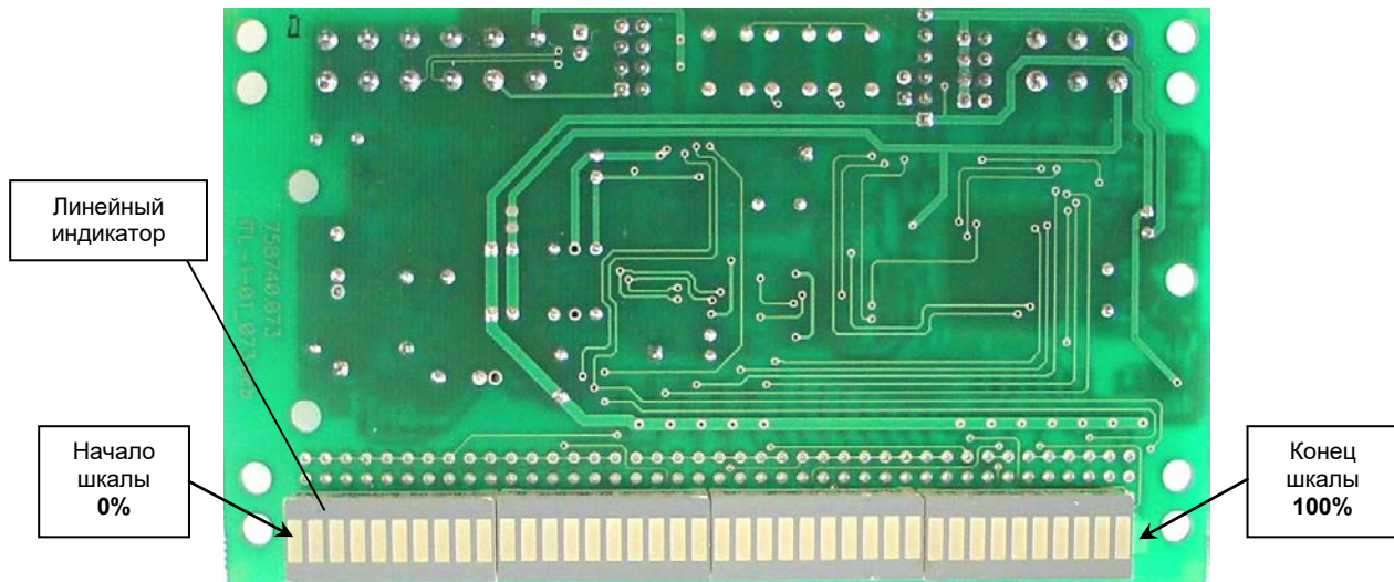
Рисунок 5.1 – Индикатор ИТМ-1-01-41. Вид спереди
