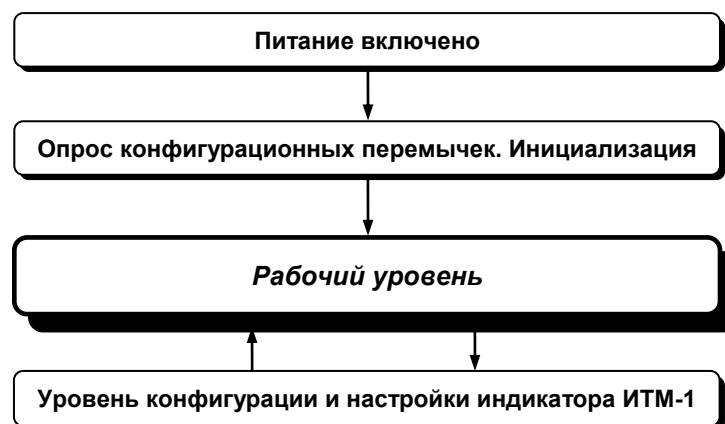
Рисунок - 6.1. Диаграмма уровней работы, конфигурации и настроек индикаторов ИТМ-1-01-31 и ИТМ-1-01-41
