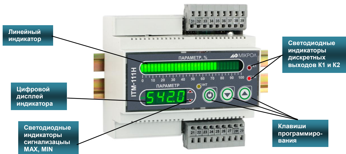
Рисунок 3.1 - Внешний вид передней панели индикатора ИТМ-111Н.
