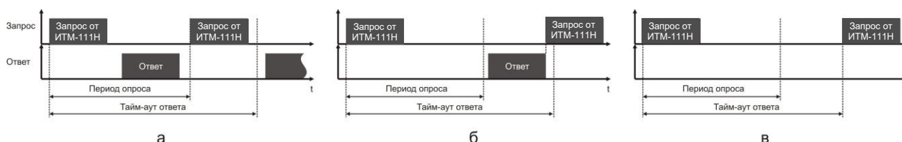
Рисунок В.3 - Временные диаграммы приема-передачи данных ИТМ-111Н в режиме MASTER
