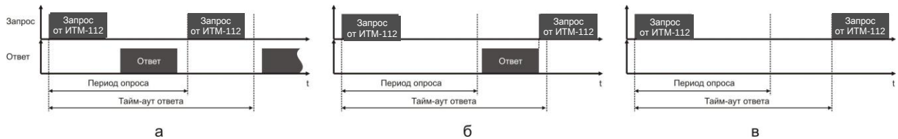
Рисунок В.2 - Временные диаграммы приема-передачи данных ИТМ-112 в режиме MASTER
