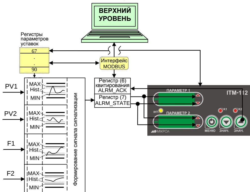
Рисунок 3.5 – Блок-схема блока сигнализации
