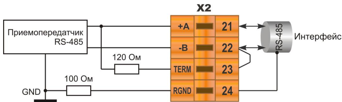
Рисунок Б.9 - Рекомендуемая схема подключения интерфейса RS-485
