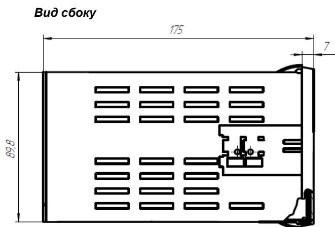
Рисунок А.1 – Внешний вид индикатора ИТМ-16
