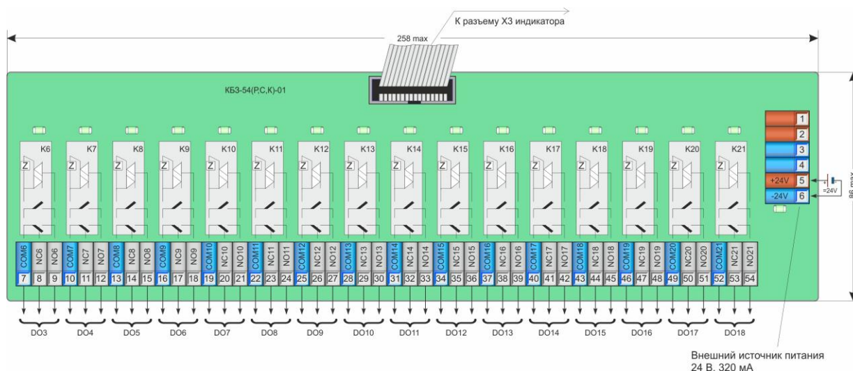
б) KB3-54P-01 с релейными дискретными выходами
