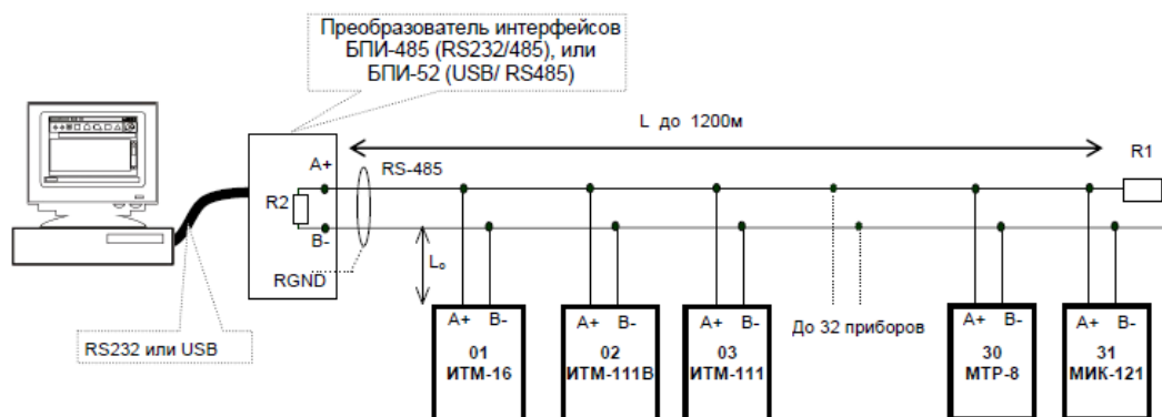
Рисунок Б.3.1 - Организация интерфейсной связи между компьютером и индикаторами или контроллерами
