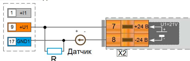
Рисунок 4.7 Подключение токового сигнала в группе аналоговых входов настроенных на сигнал от термопар
