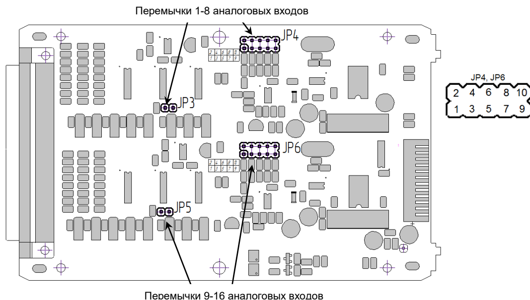
Рисунок 4.4 – Положение перемычек на плате процессора и на модуле аналогового выхода
