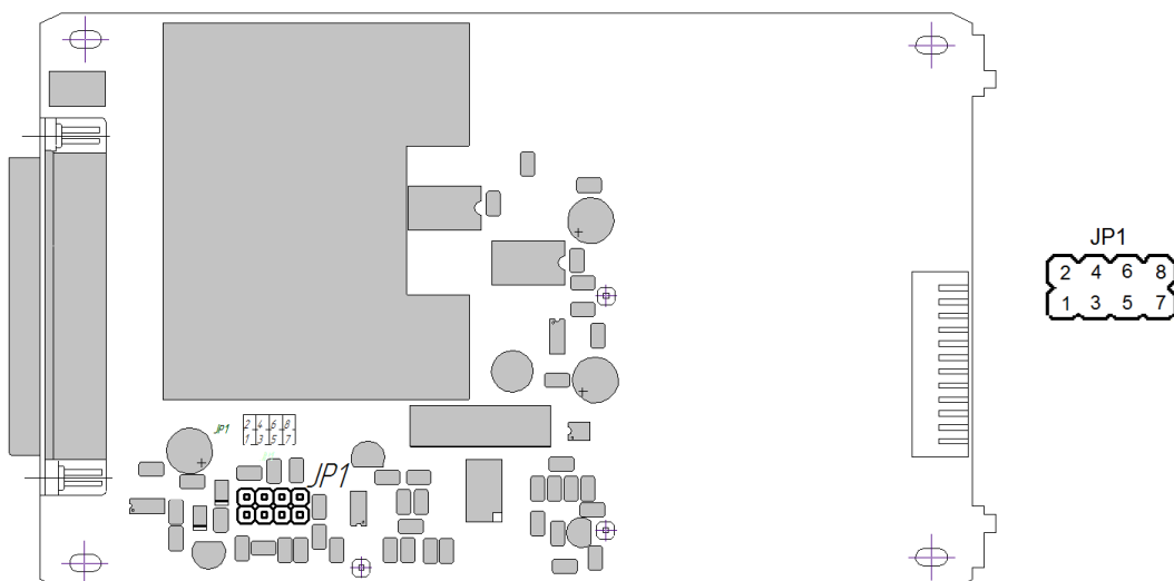
Рисунок 4.5 – Положение перемычек аналогового выхода на модуле расширения.
