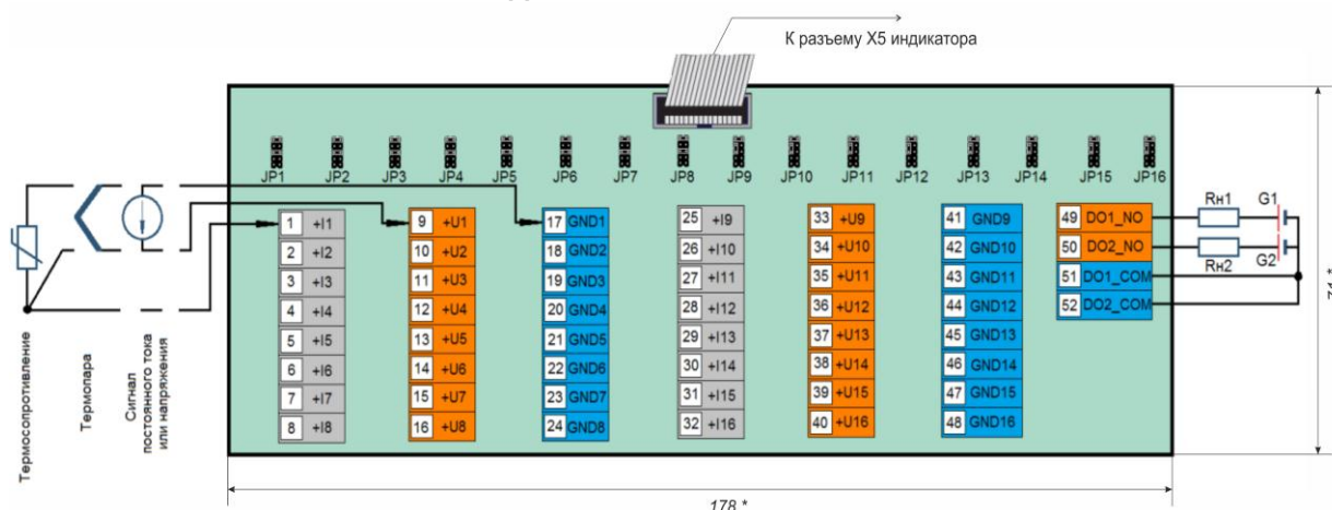
Рисунок Б.1.1 Подключение внешних цепей к индикатору ИТМ-16 через КБЗ-52-01 (разъем X5)
