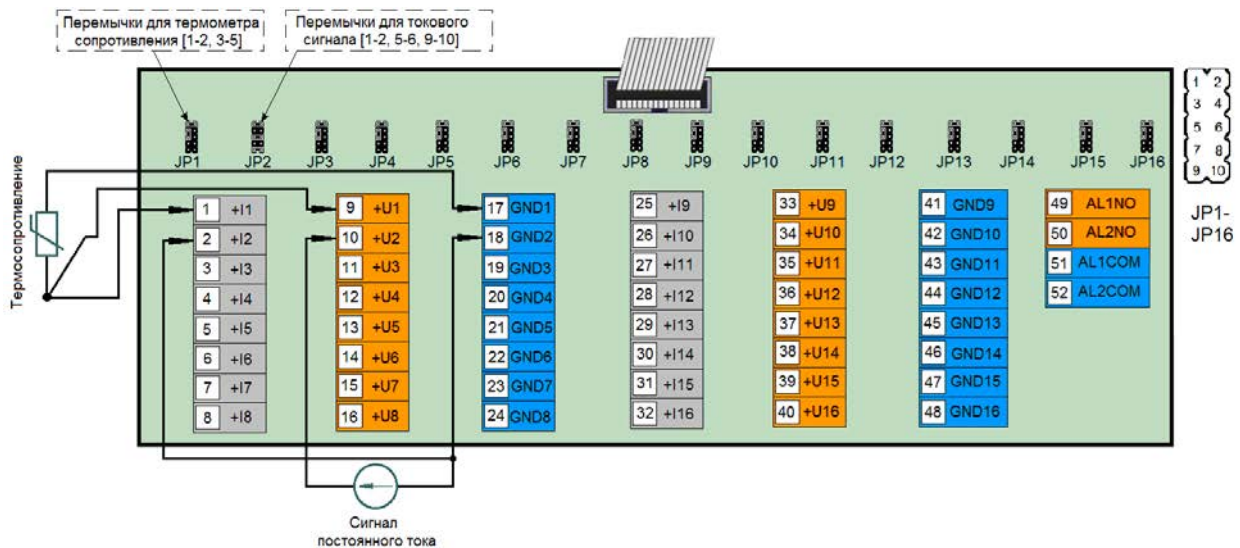
Рисунок 4.6 Подключение датчика постоянного тока (при одновременном подключении термометров сопротивления к выбранной группе аналоговых входов)
