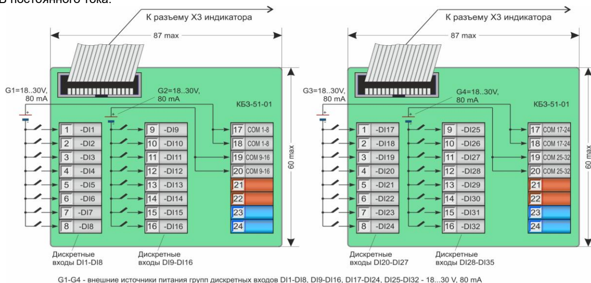
Рисунок Б.4.6 - КБ3-51-01. Схема подключения сигналов модуля расширения МР-52-30, внешний вид
