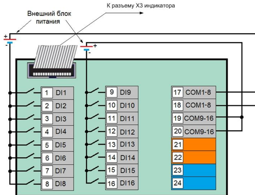
Рисунок Б.4.1 - КБЗ-24-20. Схема подключения сигналов модуля расширения МР-52-10, внешний вид
