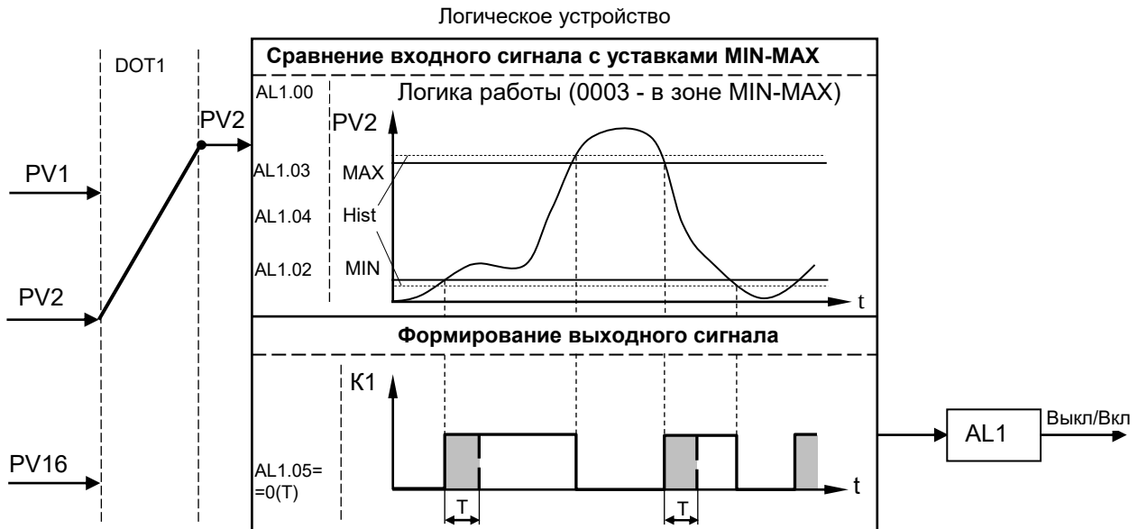
Рисунок 3.6 – Диаграмма работы логических устройств
