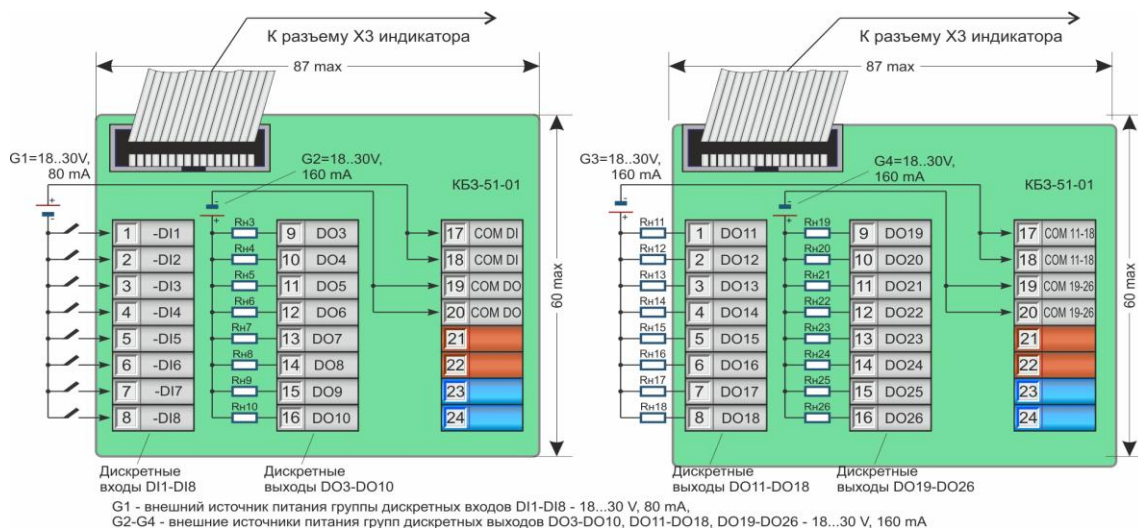
а) КБ3-51-01 с транзисторными дискретными выходами
