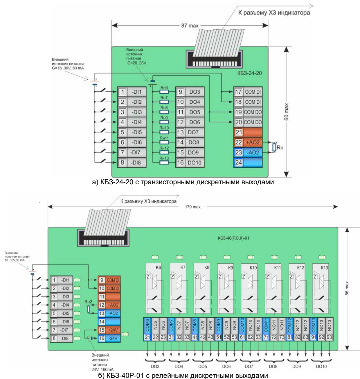
Рисунок Б.4.3 - Схема подключения сигналов модуля расширения МР-52-13, внешний вид
