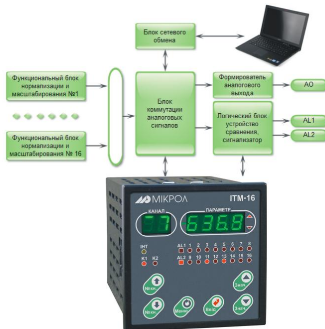
Рисунок 3.3 - Функциональная схема индикатора ИТМ-16
