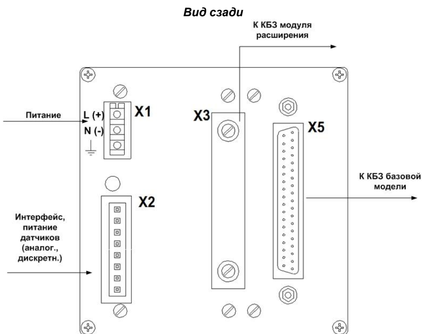
Рисунок А.2 - Габаритные размеры и назначения разъемов индикатора ИТМ-16
