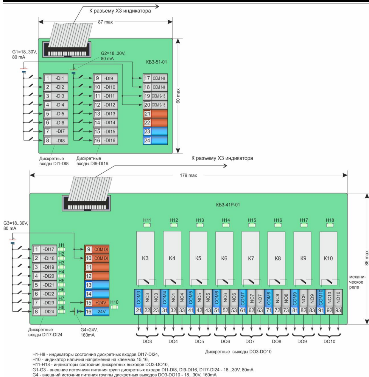
б) KB3-41P-01 с релейными дискретными выходами
