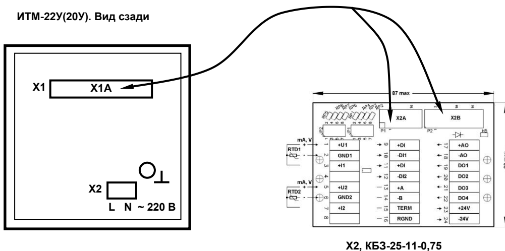
Рисунок Б.1 – Подключение клеммно-блочного соединителя KB3-25-11-0,75 к индикатору ИТМ-22У (ИТМ-20У)
