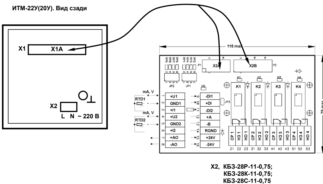
Рисунок Б.2 – Подключение клеммно-блочного соединителя к индикатору ИТМ-22У (ИТМ-20У):
