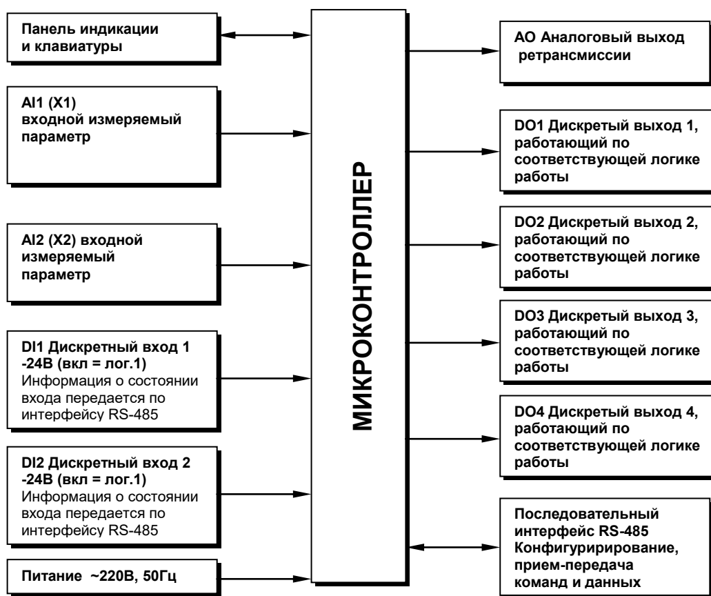
Рисунок 3.3 - Структурная схема индикатора ИТМ-22У (ИТМ-20У)
