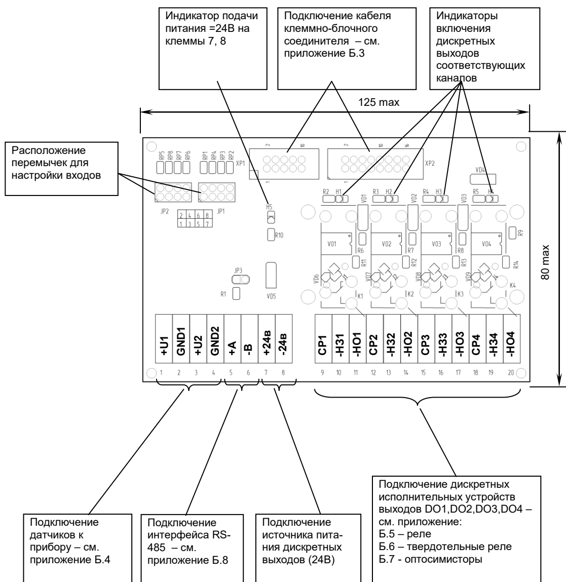
Рисунок Б.4 - Диаграмма расположения сигналов и габаритные размеры клеммно-блочных соединителей КБ3-20Р-12, КБ3-20К-12, КБ3-20С-12
