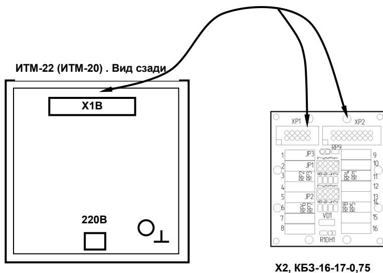
Рисунок Б.1 - Подключение клеммно-блочного соединителя КБЗ-16-17-0,75 к индикатору ИТМ-22(ИТМ-20)
