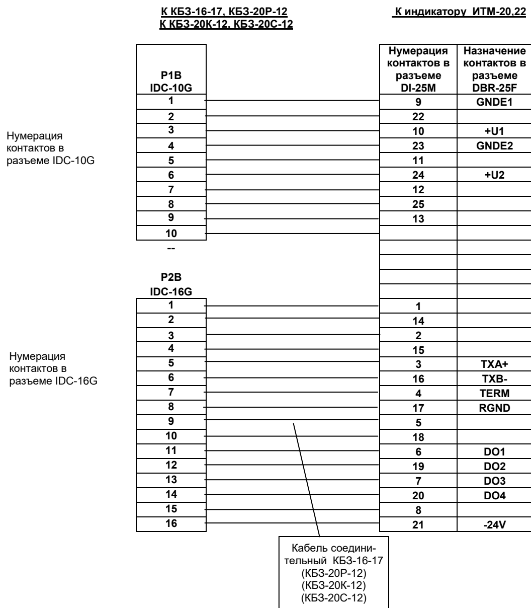
Рисунок Б.5 - Схема распайки кабеля клеммно-блочных соединителей КБЗ-16-17-0,75, КБЗ-20Р-12-0,75, КБЗ-20К-12-0,75 и КБЗ-20С-12-0,75
