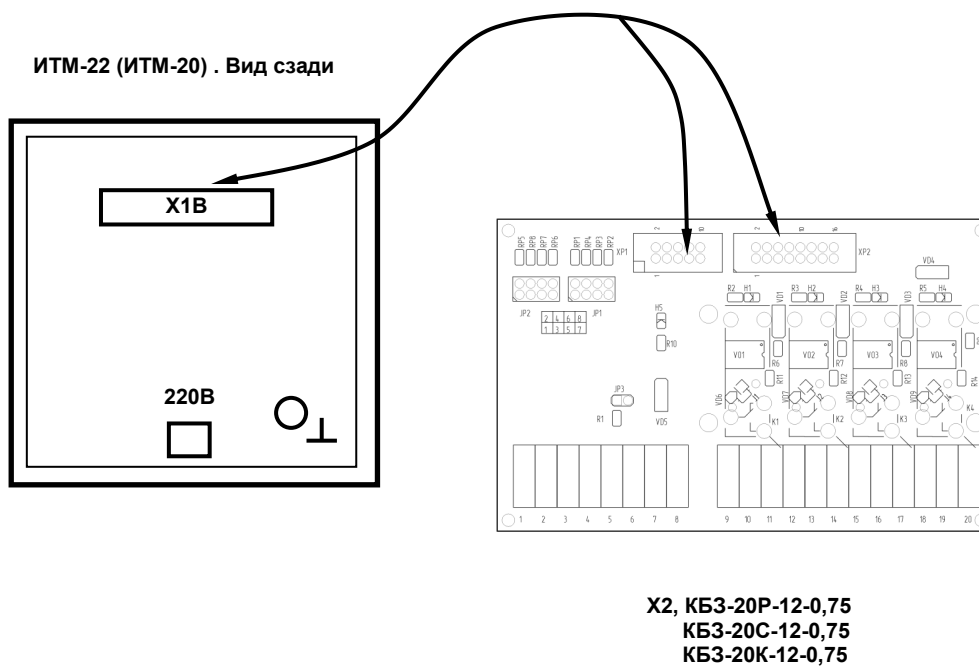
Рисунок Б.2 - Подключение клеммно-блочного соединителя к индикатору ИТМ-22(ИТМ-20): - КБЗ-20Р-12-0,75 (с реле), - КБЗ-20К-12-0,75 (с твердотельными реле), - КБЗ-20С-12-0,75 (с оптосимисторами).
