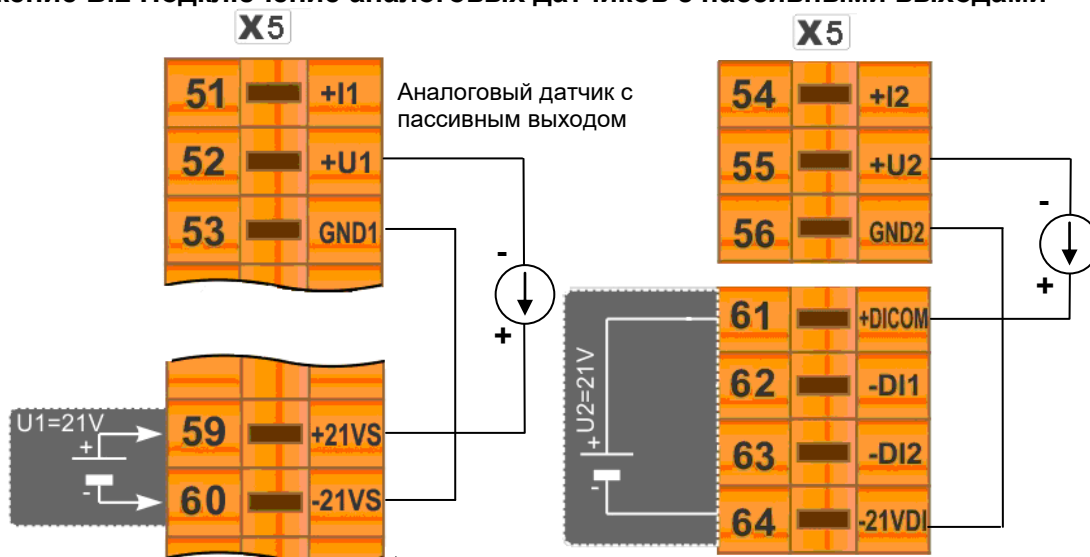
Рисунок Б.3 - Подключение к регулятору МИК-121 аналоговых датчиков с пассивными выходами
