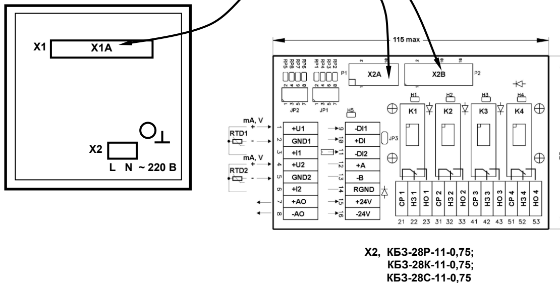
Рисунок Б.2 - Подключение клеммно-блочного соединителя - KB3-28P-11-0,75 (с реле), - KB3-28K-11-0,75 (с твердотельными реле), - KB3-28C-11-0,75 (с оптосимисторами) к регулятору МИК-22
