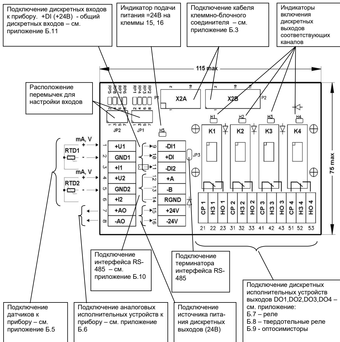
Рисунок Б.4 - Диаграмма расположения сигналов и габаритные размеры клеммно-блочных соединителей КБЗ-28Р-11, КБЗ-28К-11, КБЗ-28С-11
