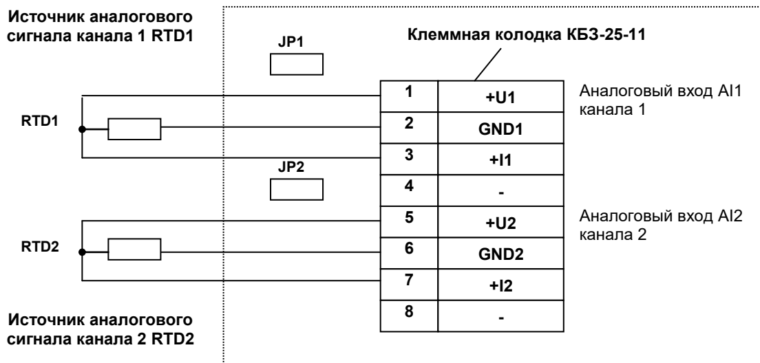
Рисунок Б.7 - Подключение датчиков температуры типа ТСМ, ТСР к аналоговым входам регулятора МИК-22
