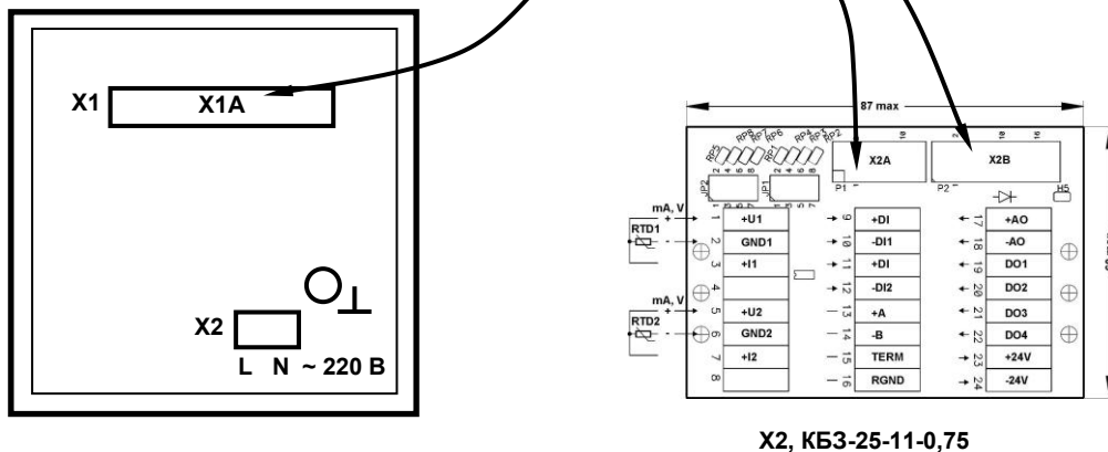
Рисунок Б.1 - Подключение клеммно-блочного соединителя KB3-25-11-0,75 к регулятору МИК-22
