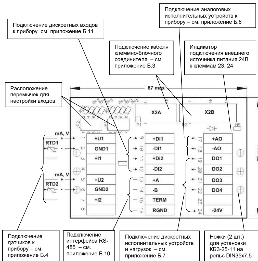
Рисунок Б.3 - Схема расположения сигналов и габаритные размеры клеммно-блочного соединителя КБЗ-25-11
