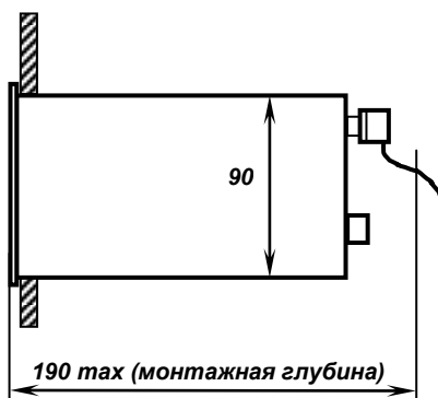
Рисунок А.2 - Габаритные размеры
