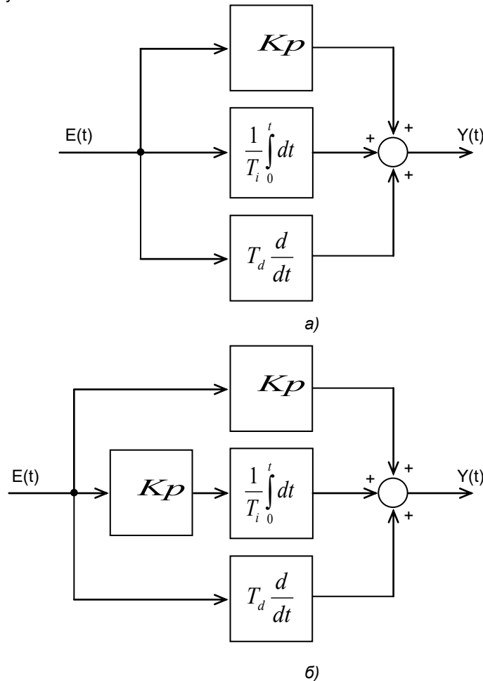
Рисунок 10.2 – Структуры регуляторов МИК-22
